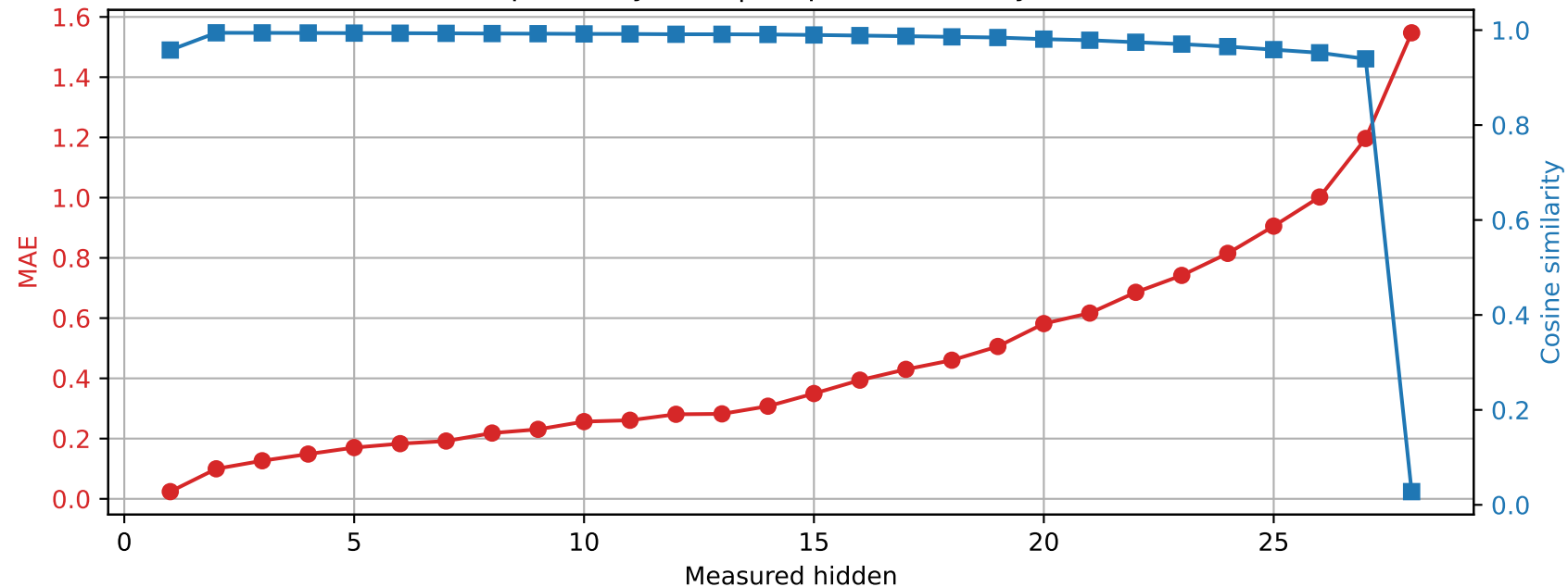
Llama-3.2-3B | Prompt 4 Spared layer 19 | Unquantized vs hybrid
