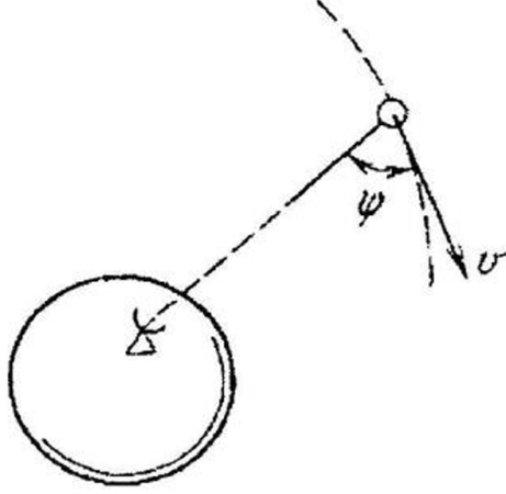
Рис. 1.4. Схема для расчета доплеровского смещения
