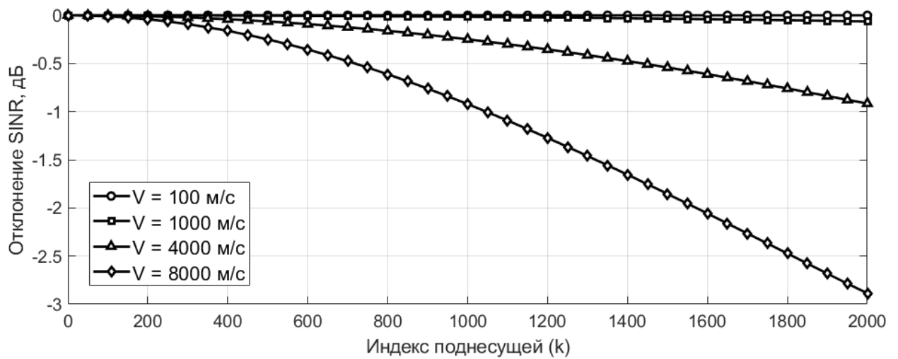
Рис. 1.5. Зависимость отклонения SINR от k в отсутствии доплеровского сдвига несущей частоты
