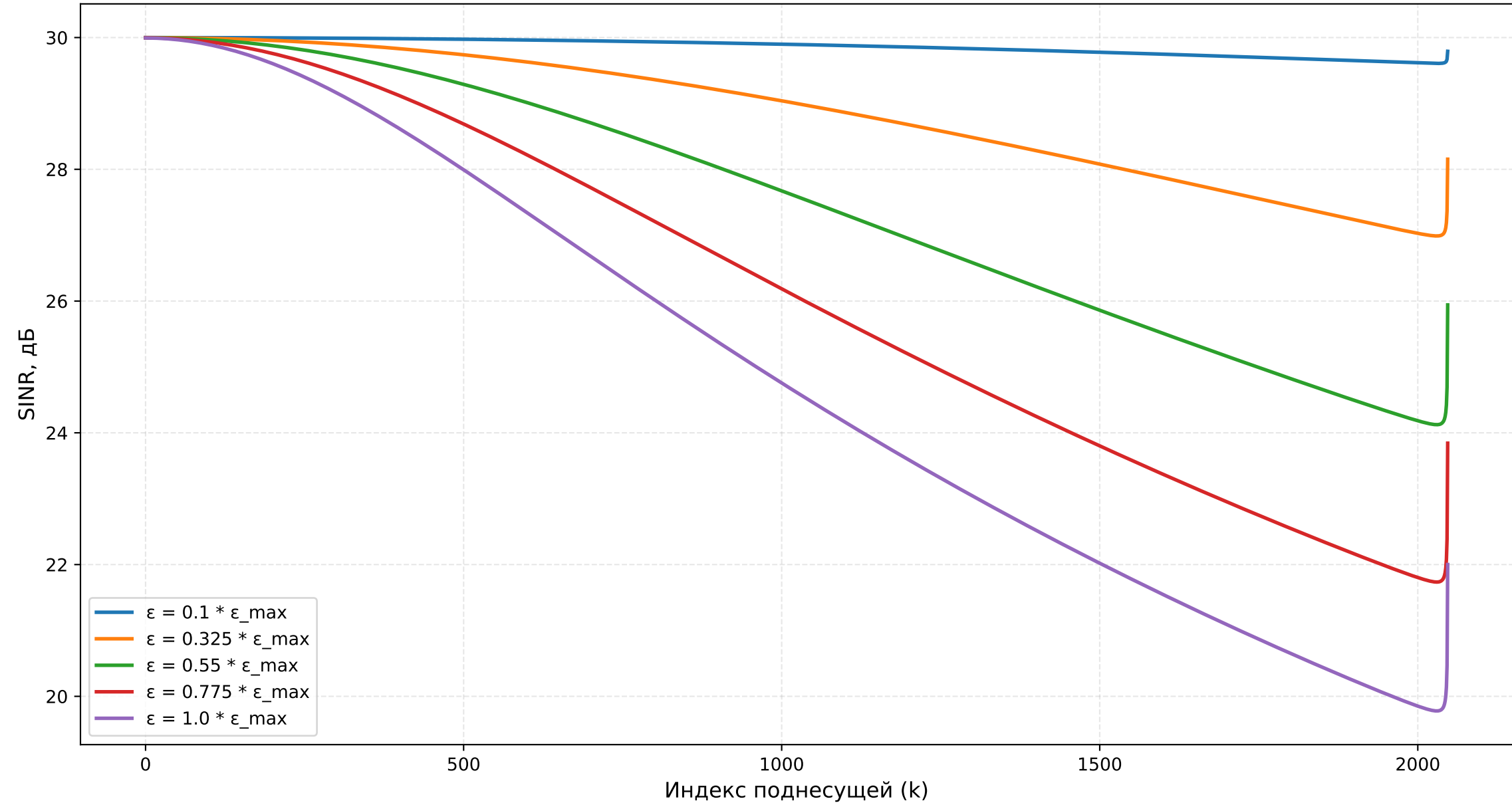
Теоретический SINR для OFDM системы (N=2048, SNR=30 дБ)
