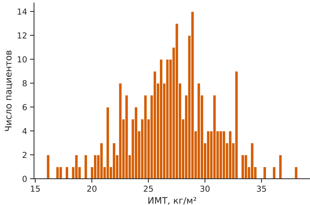
Плохо: слишком много бинов (80)
