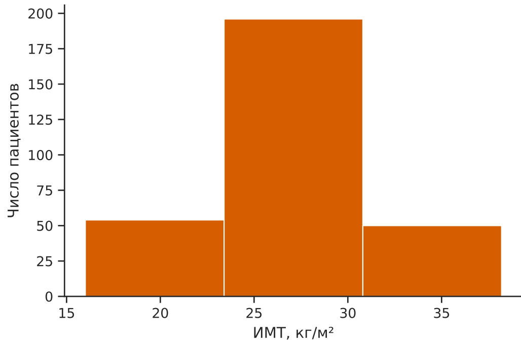
Плохо: слишком мало бинов (3)
