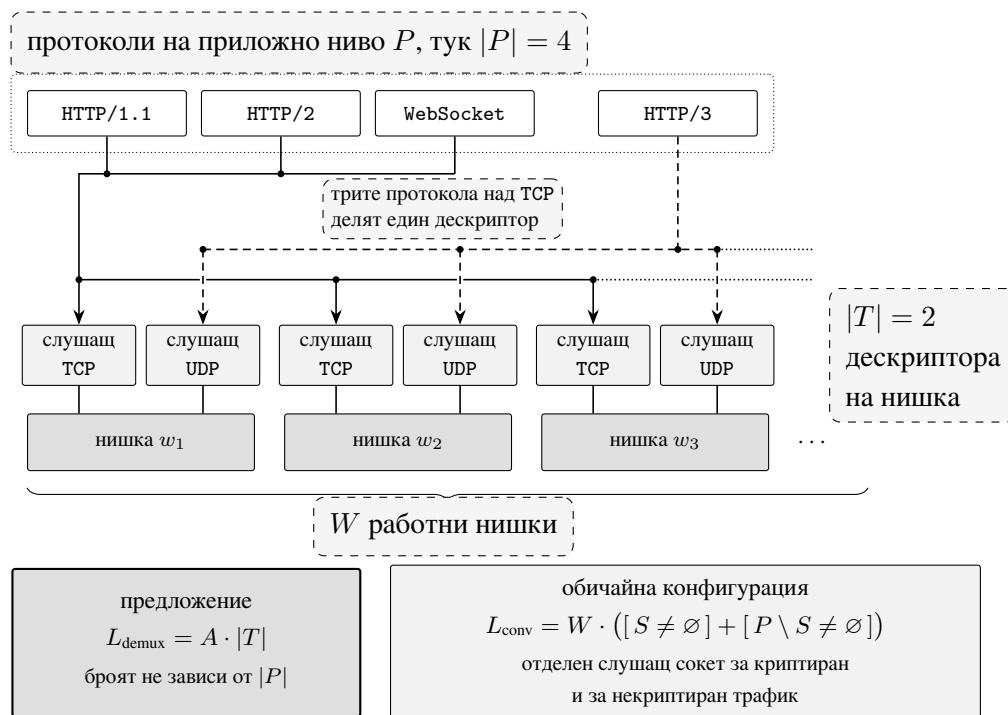
Фигура 3. Брой на слушащите дескриптори при класификация след приемане на връзката.
