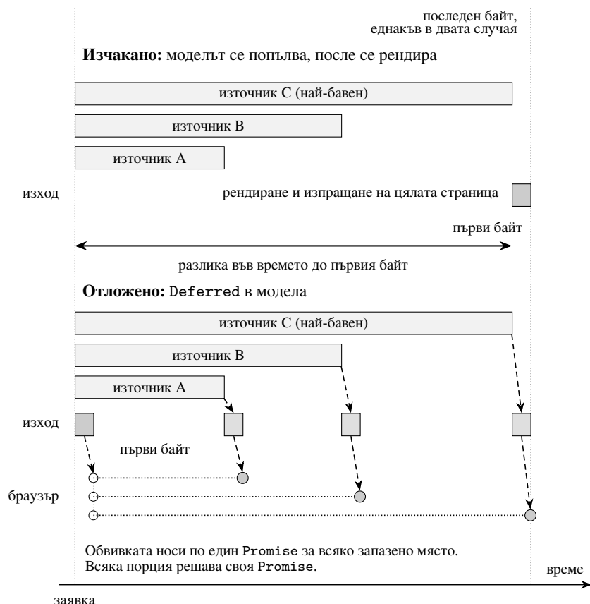
Фигура 8. Изчакано и отложено рендиране върху обща времева ос. Горے моделът се попълва изцяло, преди да тръгне какъвто и да е байт, затова първият байт съвпада с края на най-бавната заявка. Долу обвивката на страницата тръгва веднага, със запазени места, а всяка стойност пътува като отделна порция, щом пристигне. Последният байт е на едно и също място в двата случая, защото и в двата се определя от най-бавната заявка. Спестява се време до първия байт, а не общо време.
