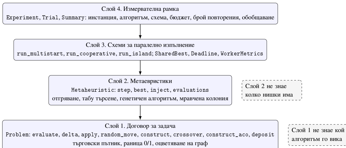
Фигура 1. Слоеви и посока на зависимостите
