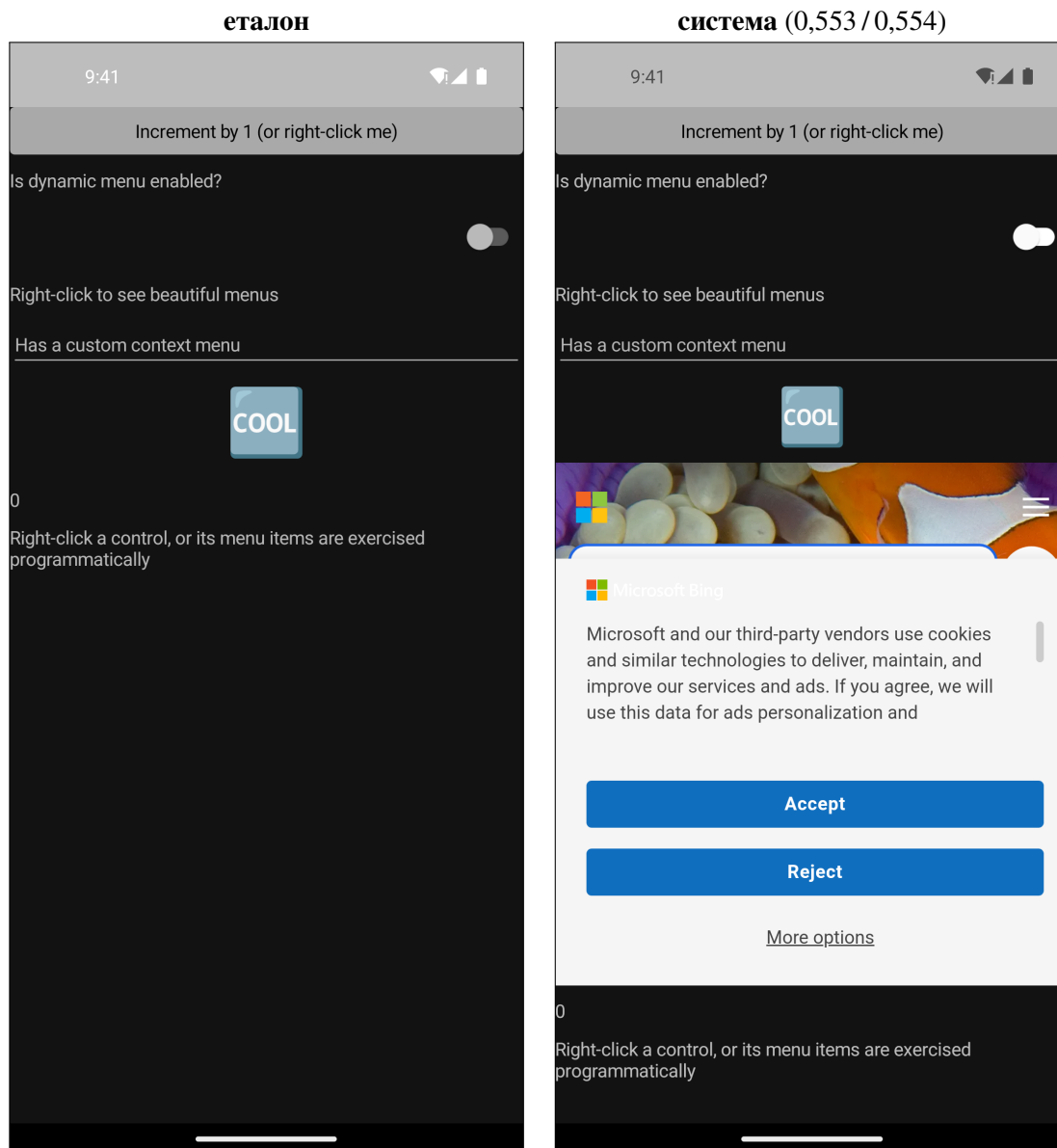
Фигура 18. context_flyout — Android, тъмна тема. Структурно сходство 0,553 по код и 0,554 от описанието. Живо външно уеб съдържание.
