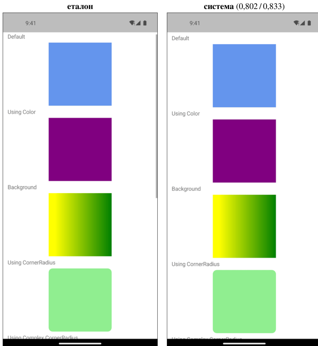
Фигура 27. box_view — Android, светла тема. Структурно сходство 0,802 по код и 0,833 от описанието. Открит.
