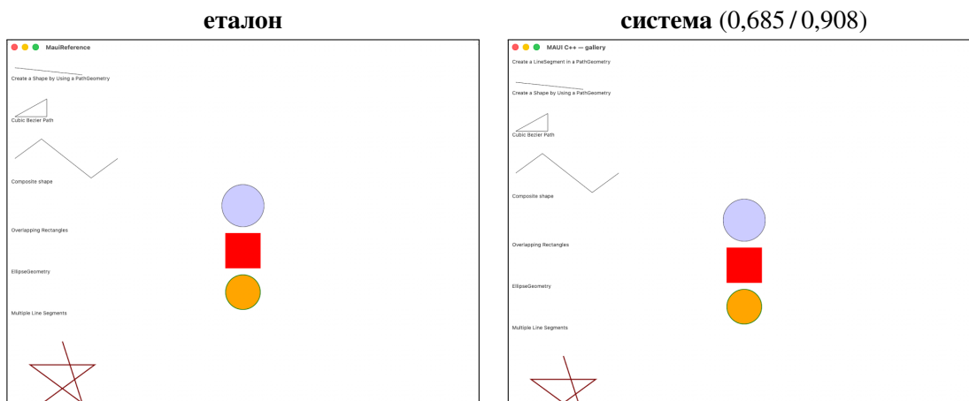
Фигура 22. path_gallery — Mac Catalyst, светла тема. Структурно сходство 0,685 по код и 0,908 от описанието. Открит.
