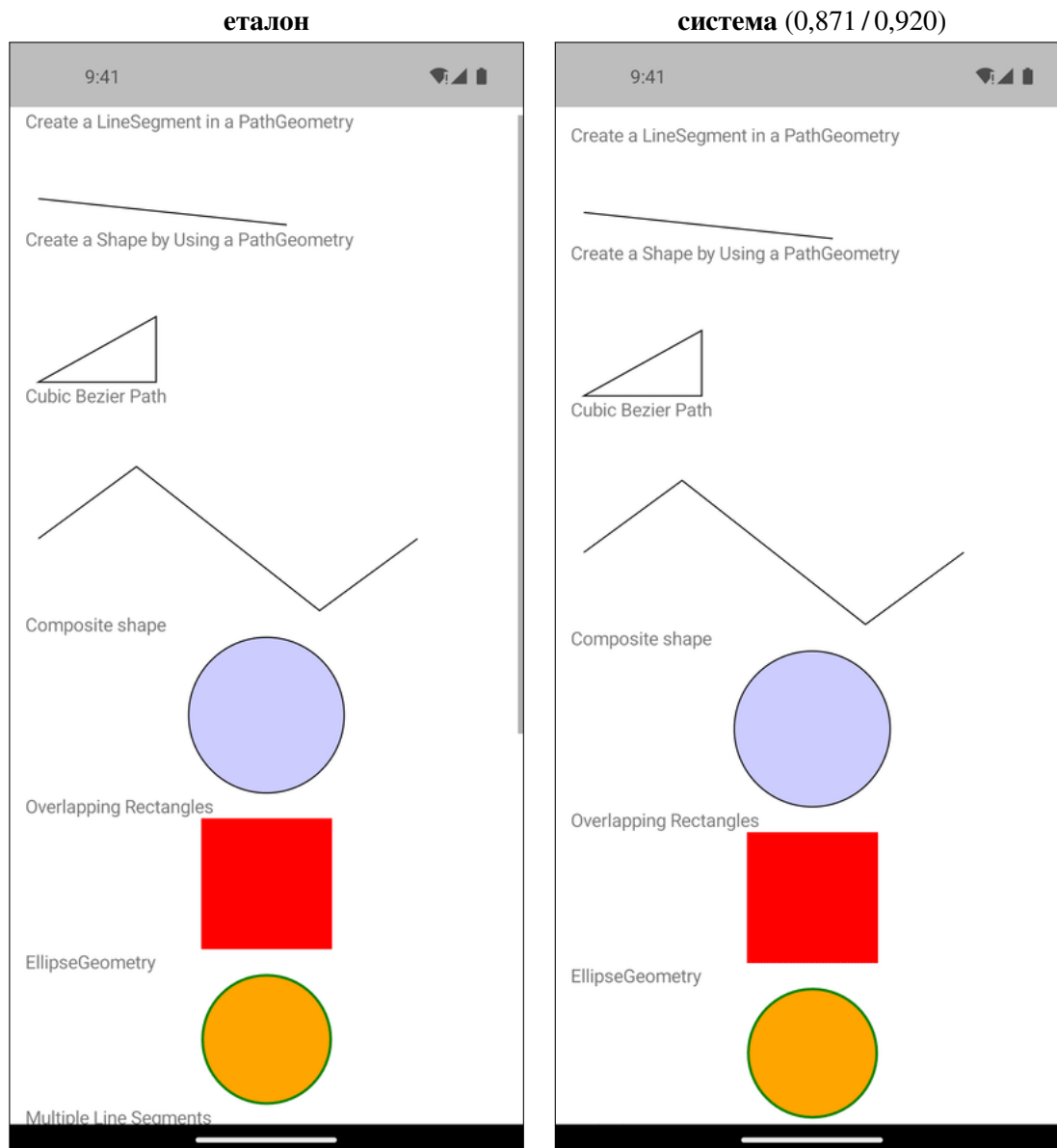
Фигура 29. path_gallery — Android, светла тема. Структурно сходство 0,871 по код и 0,920 от описанието. Открит.
