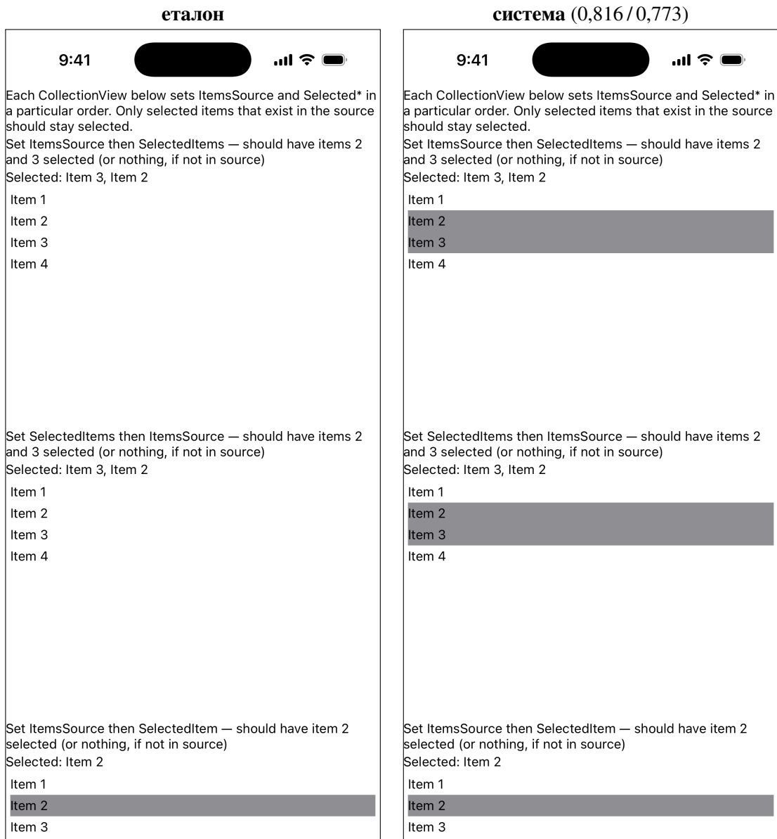
Фигура 25. selection_synchronization — iOS, светла тема. Структурно сходство 0,816 по код и 0,773 от описанието. Открит.
