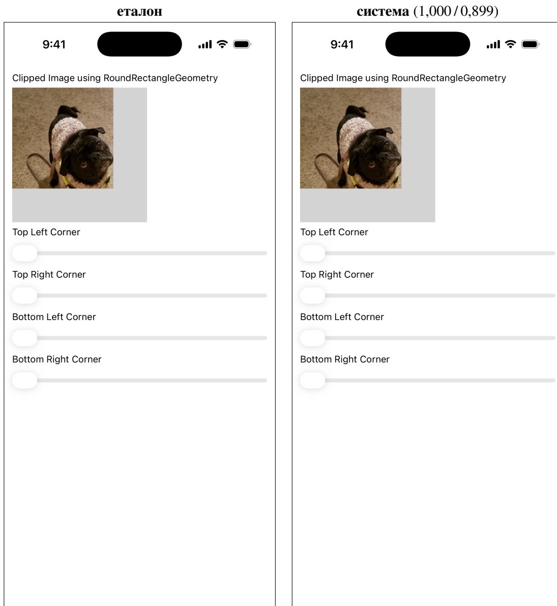
Фигура 31. clip_corner_radius — iOS, светла тема. Структурно сходство 1,000 по код и 0,899 от описанието. Открит.
