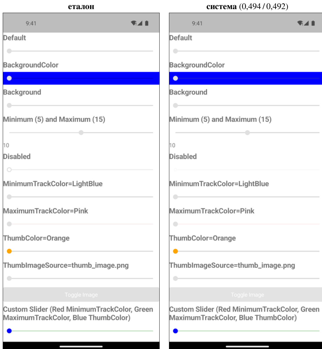
Фигура 17. slider — Android, светла тема. Структурно сходство 0,494 по код и 0,492 от описанието. Открит.
