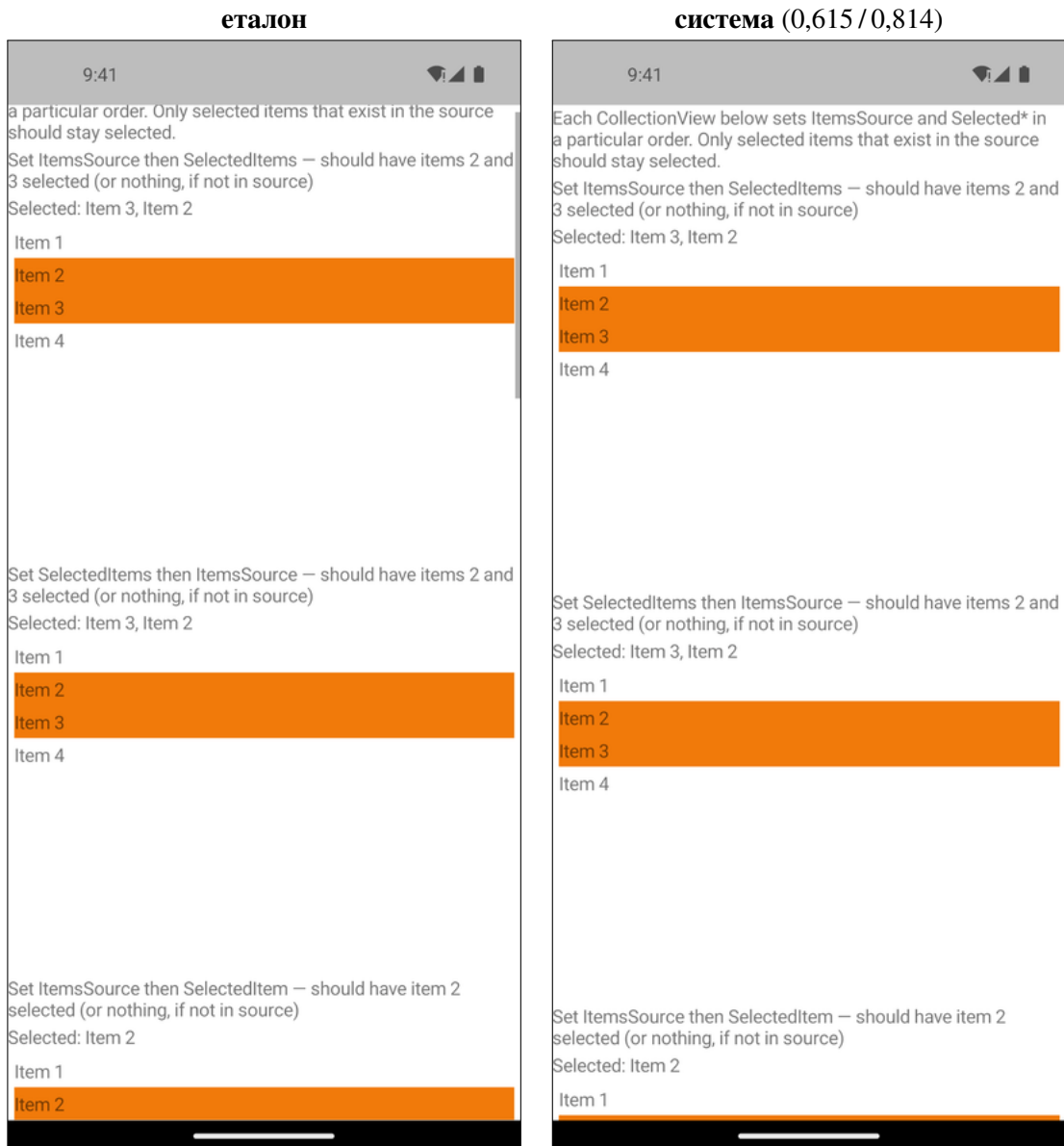
Фигура 19. selection_synchronization — Android, светла тема. Структурно сходство 0,615 по код и 0,814 от описанието. Открит.
