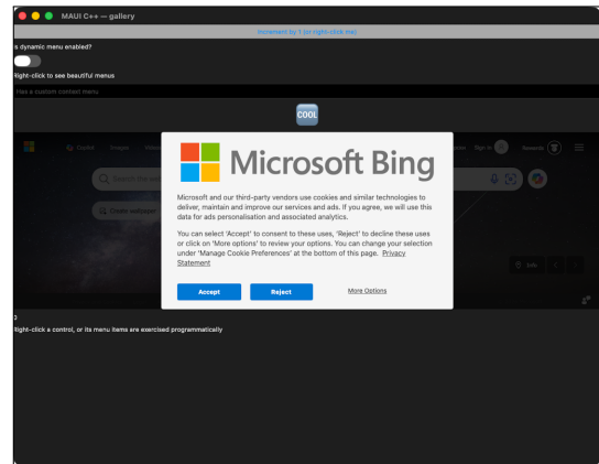
система (0,853/0,915)
