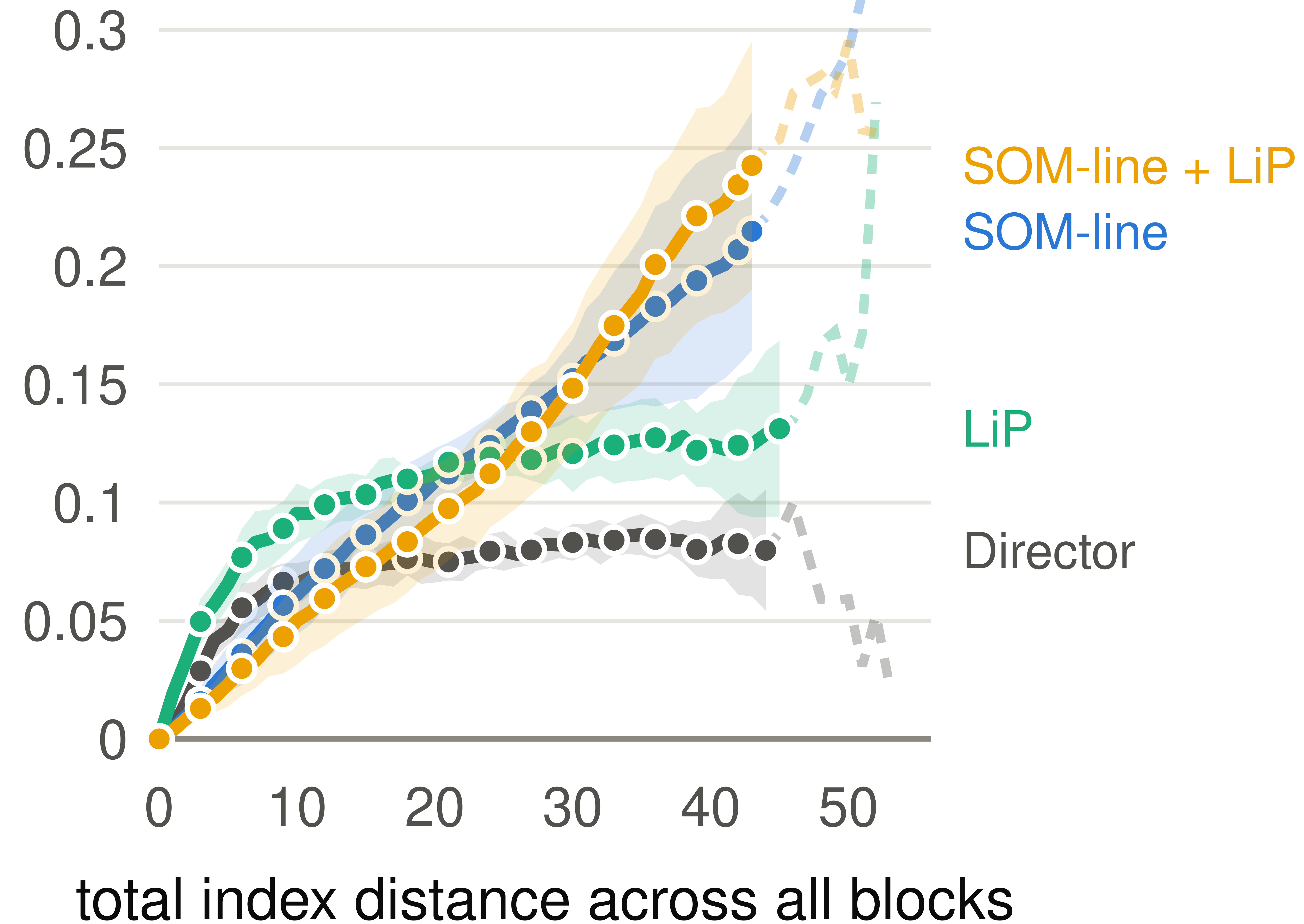
Hopper Stand
