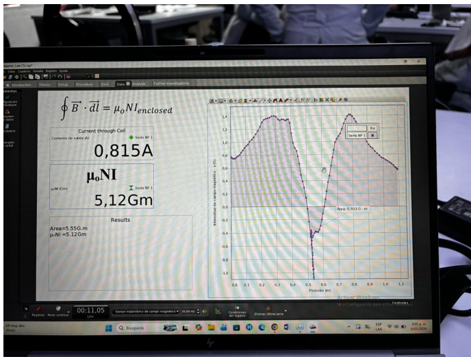
Figura 8: Recorrido 2 (rodea el exterior): regiones positivas y negativas que casi se cancelan; área = 0,933 G·m \approx 0 .
