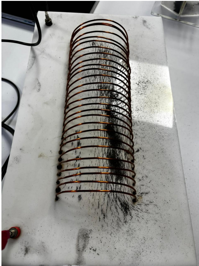
Figura 2: Solenoide con limadura de hierro. Las líneas emergen por un extremo y se cierran por el otro, igual que en un imán de barra.
