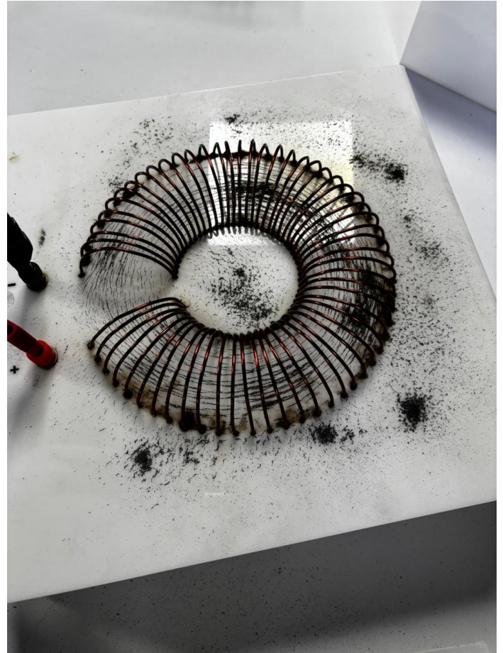
Figura 1: Toroide con limadura de hierro. Las líneas de campo quedan completamente confinadas dentro del núcleo toroidal, sin flujo en el exterior.
