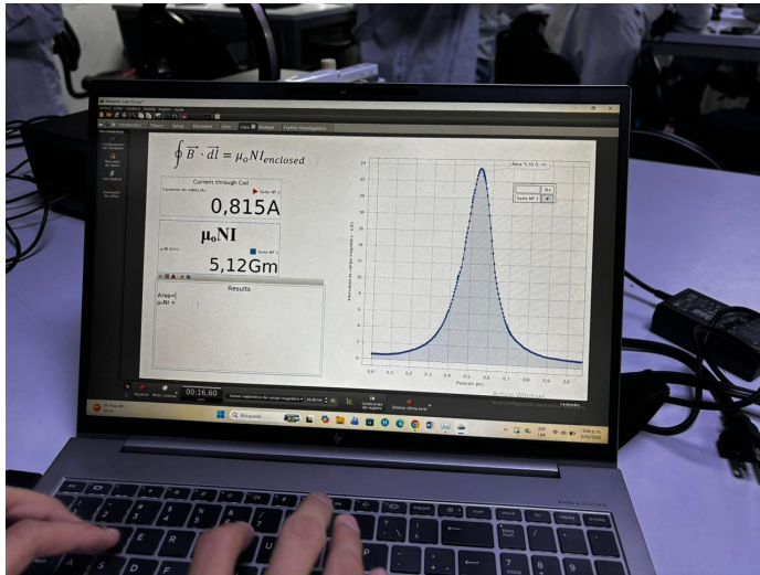
Figura 7: Recorrido 1 (por el centro): pico tipo campana, área = 5,55 G·m \approx \mu_0 N I = 5,12 Gm. I = 0,815 A.
