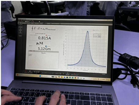
Figura 7: Recorrido 1 (por el centro): pico tipo campana, área = 5,55\text{ G·m} \approx \mu_0 NI = 5,12\text{ Gm} . I = 0,815\text{ A} .
