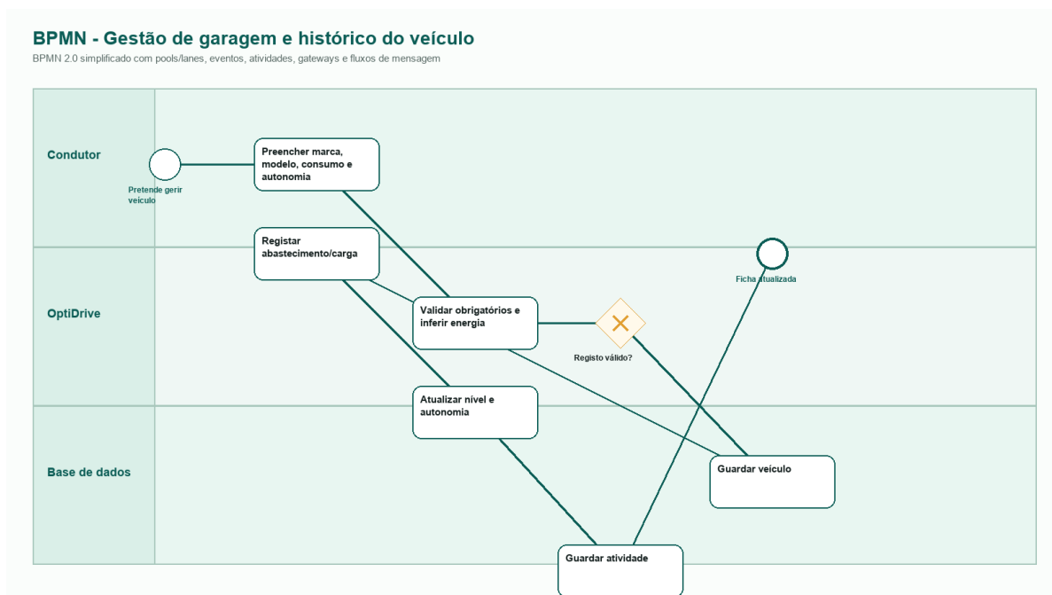
Figura 2 - BPD da Sprint 1.
