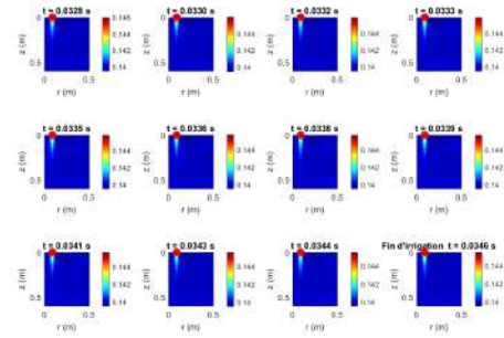
FIG. 4.2 : Évolution spatio-temporelle de la teneur en eau et progression du front d'irrigation jusqu'à la fin de l'irrigation pour la culture du maïs dans un sol sableux.
