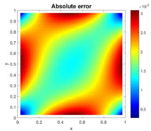
FIG. 2.14 : Erreur pour h = 0.04
