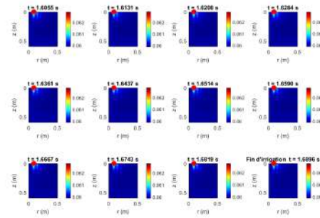
FIG. 4.6 : Évolution spatio-temporelle de la teneur en eau et progression du front d'irrigation jusqu'à la fin de l'irrigation pour la culture du coton dans un sol sableux.
