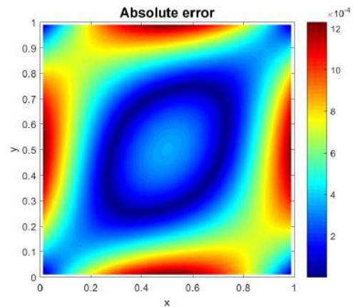
FIG. 2.16 : Erreur pour h = 0.01
