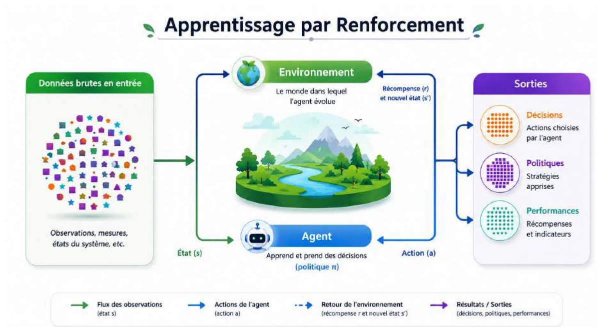
FIG. 2.23 : Architecture générale d'un système d'apprentissage par renforcement.
