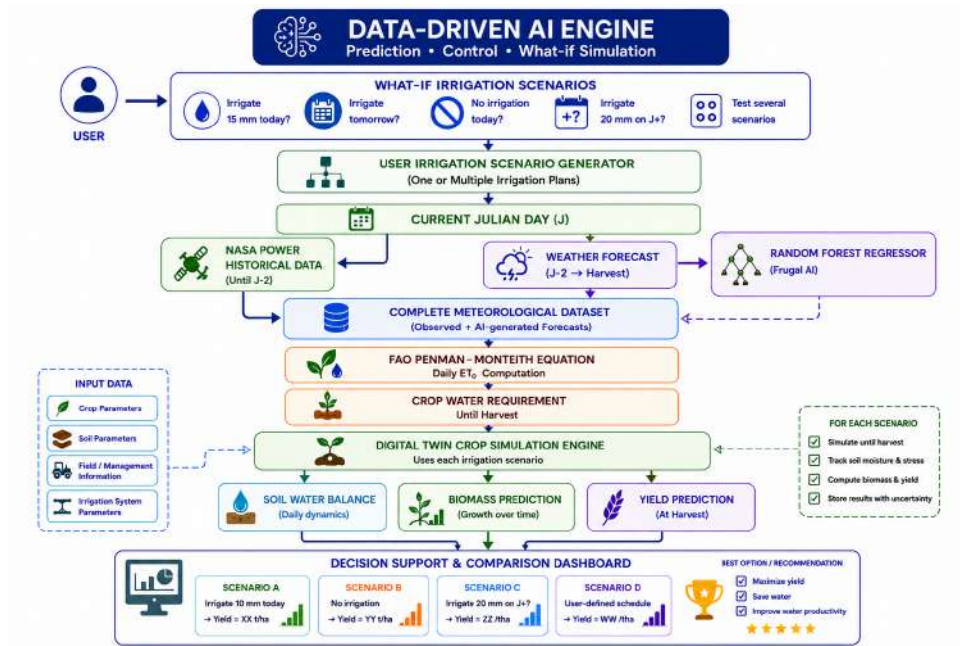
FIG. 3.7 : Fonctionnement du moteur Data-Driven AI.
