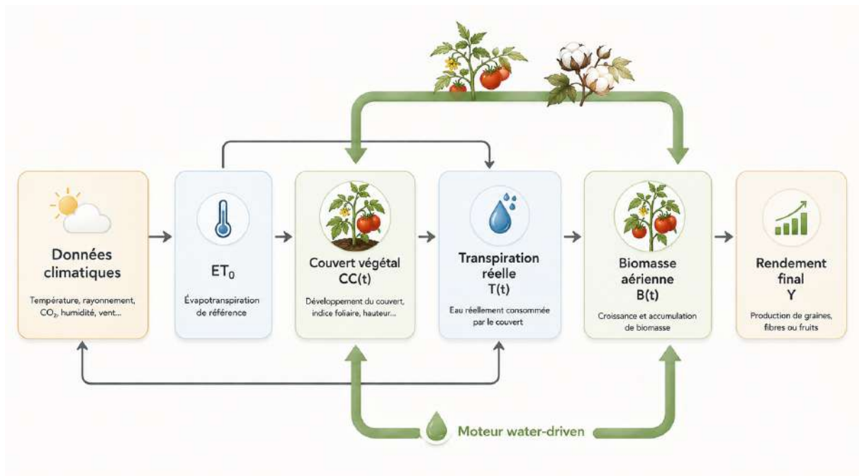
FIG. 2.18 : Flux du moteur de croissance water-driven d'AquaCrop. La séquence débute par le calcul de l'évapotranspiration de référence ET_0 à partir des données climatiques, puis détermine la transpiration réelle en fonction du couvert végétal et des stress hydriques. La biomasse est ensuite calculée via le paramètre conservatif WP^* (productivité de l'eau normalisée), et le rendement final est obtenu par application de l'indice de récolte HI .
