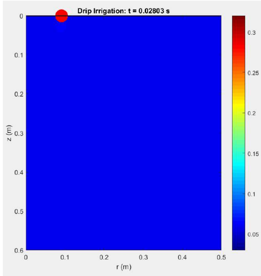
FIG. 4.7 : Évolution du bulbe d'humectation dans le cadre du test de comparaison.
