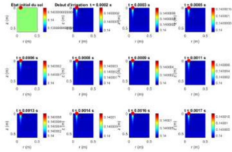
FIG. 4.1 : Évolution spatio-temporelle de la teneur en eau et progression du front d'irrigation au début de l'irrigation pour la culture du maïs dans un sol sableux.
