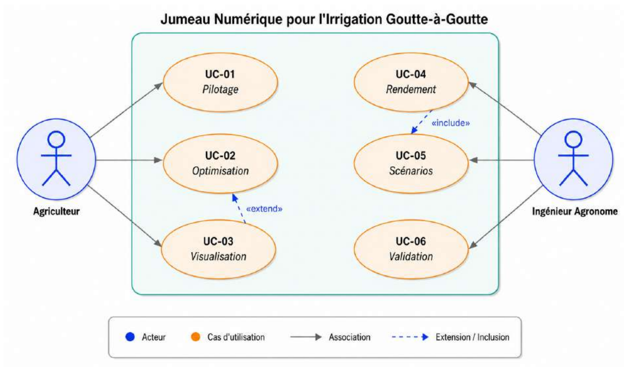
FIG. 2.2 : Diagramme de cas d'utilisation du jumeau numérique.
