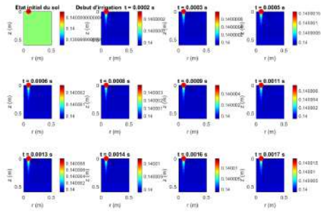
FIG. 4.3 : Évolution spatio-temporelle de la teneur en eau et progression du front au début de l'irrigation pour la culture de la tomate dans un sol sableux.
