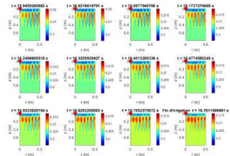
FIG. 4.13 : Évolution spatio-temporelle de la teneur en eau et progression du front d'irrigation jusqu'à la fin de l'irrigation pour la culture de la tomate dans un sol sableux avec des données Open Meteo pour une localisation définie par 6.4 (latitude) ; 2.09 (longitude).
