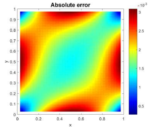
FIG. 2.12 : Erreur pour h = 0.1
