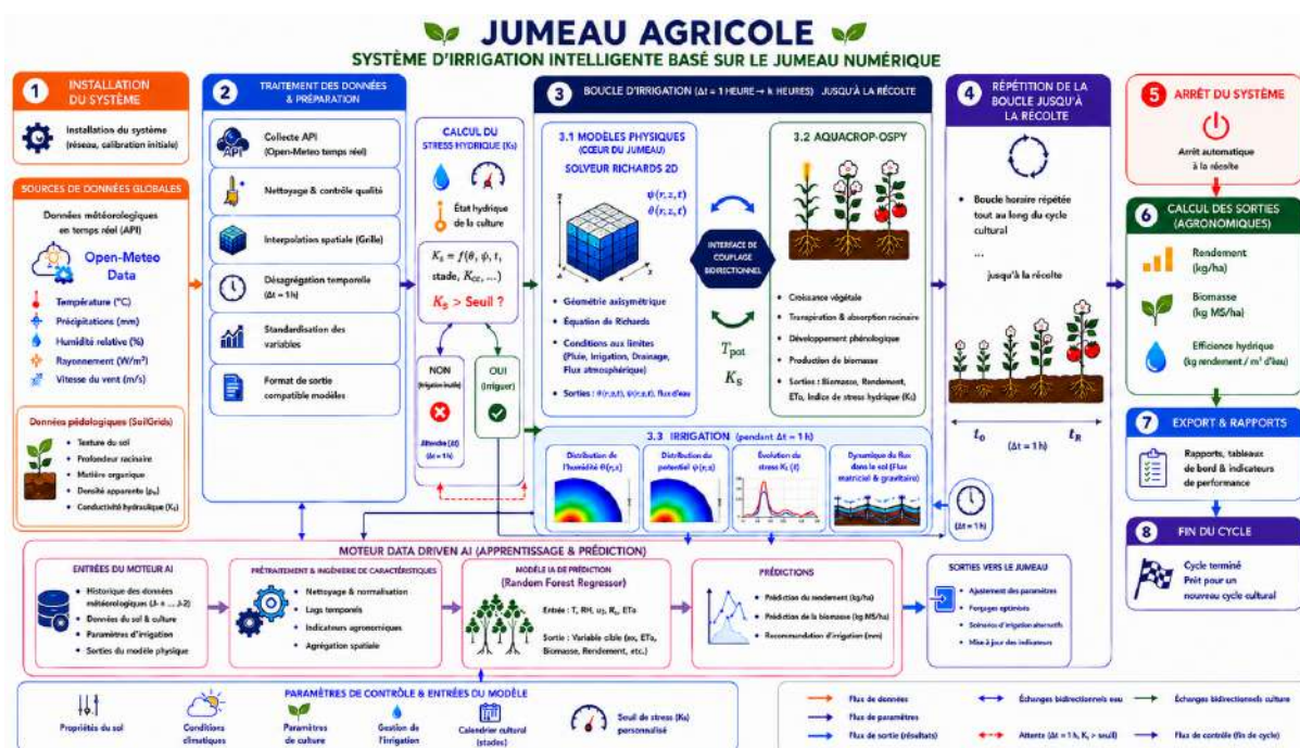
FIG. 3.3 : Architecture technique du système
