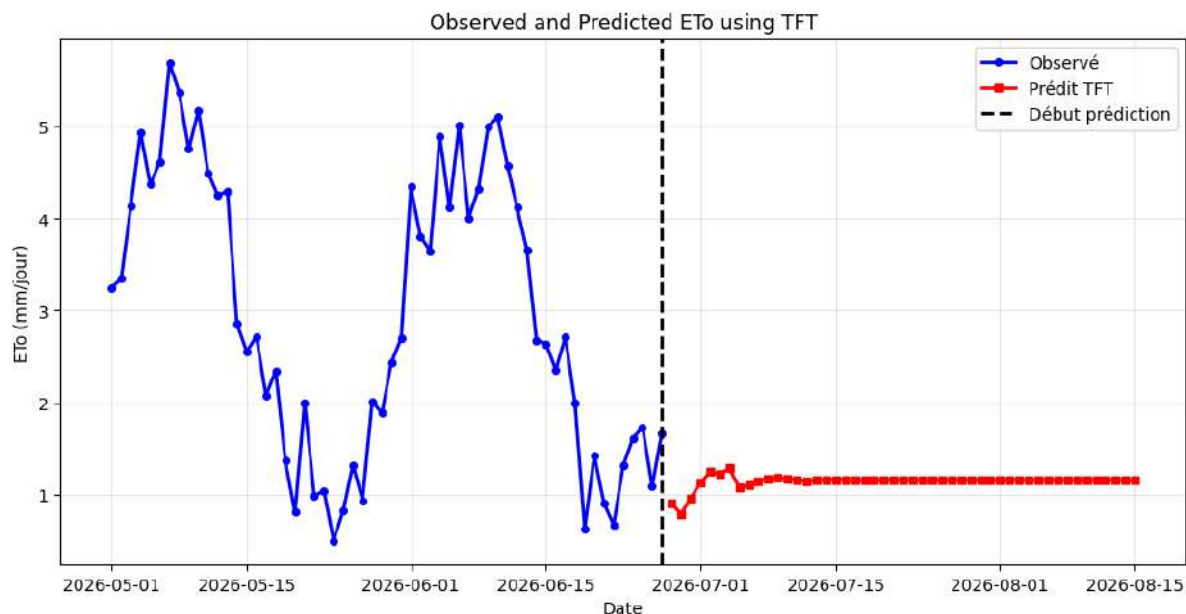
FIG. 4.21 : Prédiction de l'évapotranspiration avec TFT (Temporal Fusion Transformer).
