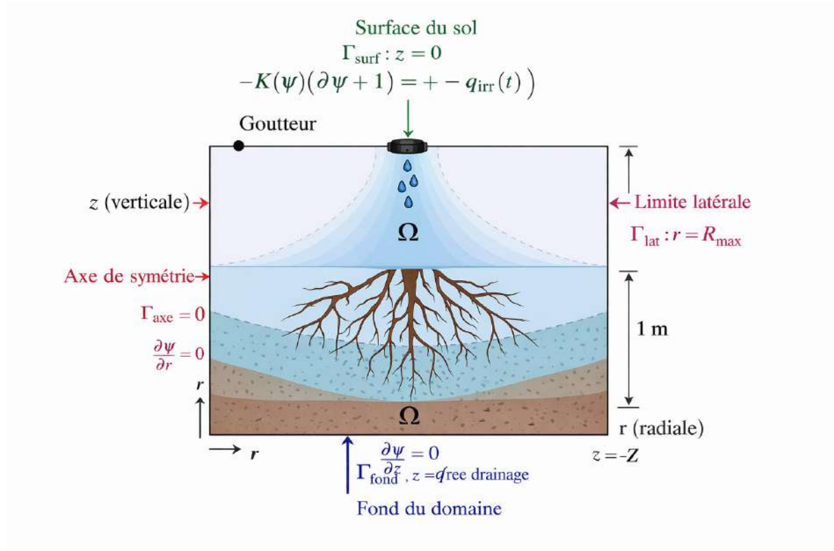
FIG. 1.19 : Domaine de simulation axisymétrique et conditions aux limites appliquées à l'équation de Richards pour l'irrigation goutte-à-goutte.
