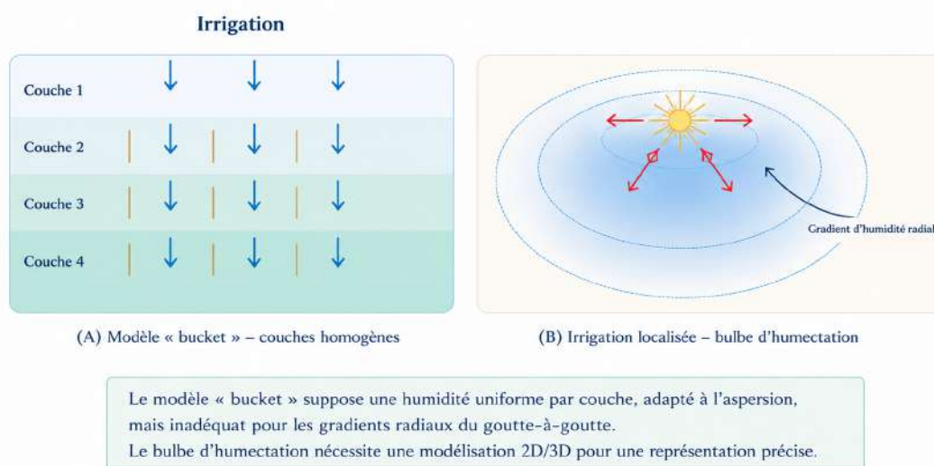
FIG. 1.5 : Comparaison schématique entre le modèle en couches homogènes « bucket » et la distribution hétérogène d'humidité sous irrigation goutte-à-goutte (bulbe d'humectation).
