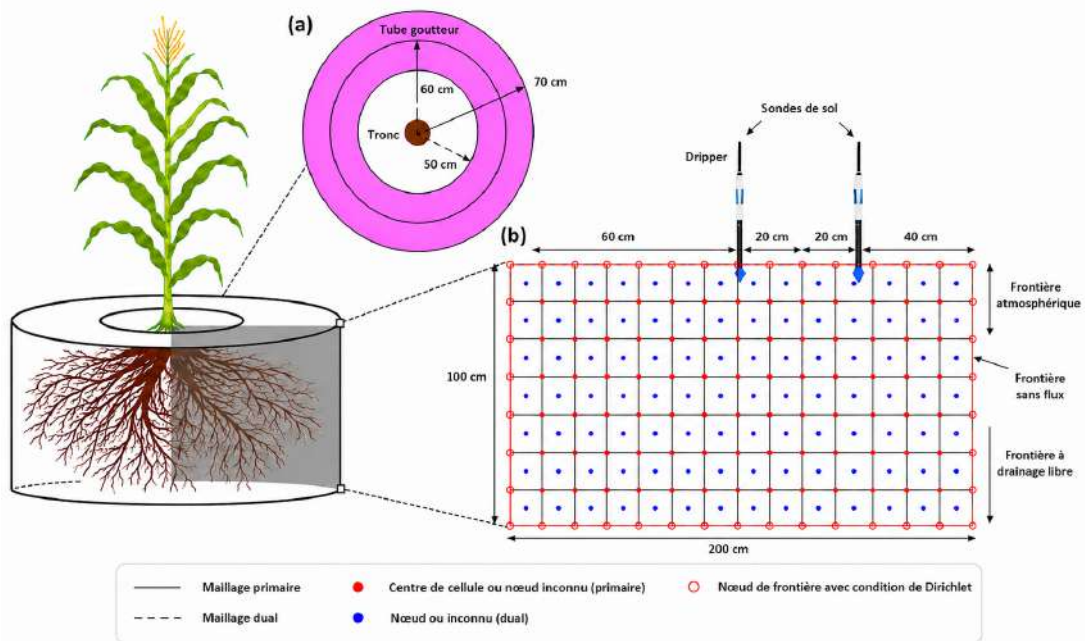
FIG. 1.18 : Configuration du domaine de simulation pour l'irrigation goutte-à-goutte : géométrie axisymétrique, conditions aux limites et maillage primal-dual.
