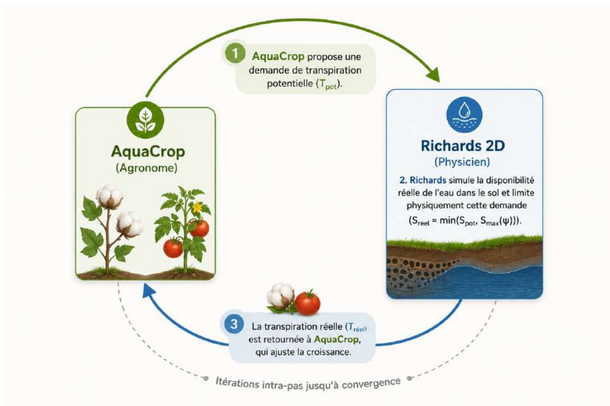
FIG. 2.17 : Schéma du couplage bidirectionnel fort entre AquaCrop et le solveur Richards. AquaCrop propose une demande, et Richards la limite physiquement via des itérations intra-journalières jusqu'à convergence.
