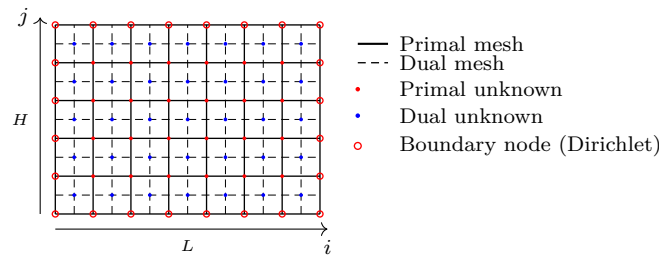
FIG. 2.5 : Maillage volumes finis en dualité discrète.
