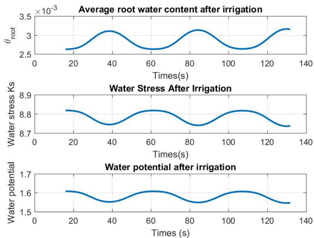
FIG. 4.14 : Évolution temporelle des indicateurs hydriques après irrigation précédente pour le maïs (teneur en eau moyenne racinaire, stress hydrique et potentiel hydrique)
