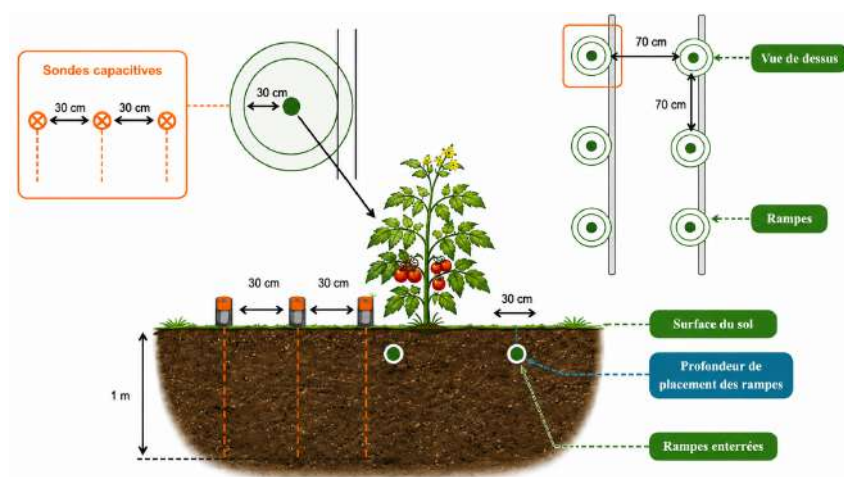
FIG. 1.2 : Montage expérimental pour l'installation d'une rampe d'irrigation et de sondes capacitatives
