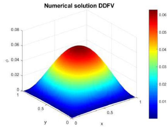
FIG. 2.11 : Solution numérique pour h = 0.01
