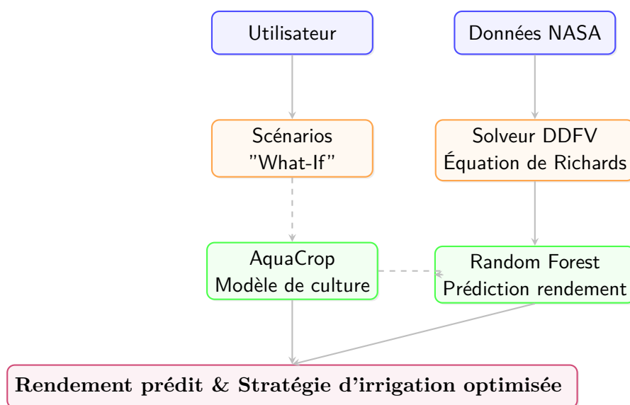
FIG. 2.1 : Architecture du jumeau numérique pour l'irrigation goutte-à-goutte
