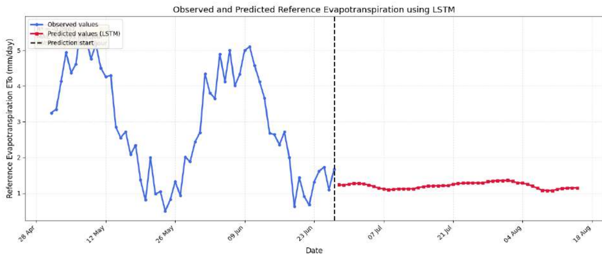
FIG. 4.20 : Prédiction de l'évapotranspiration avec LSTM (Long Short-Term Memory).
