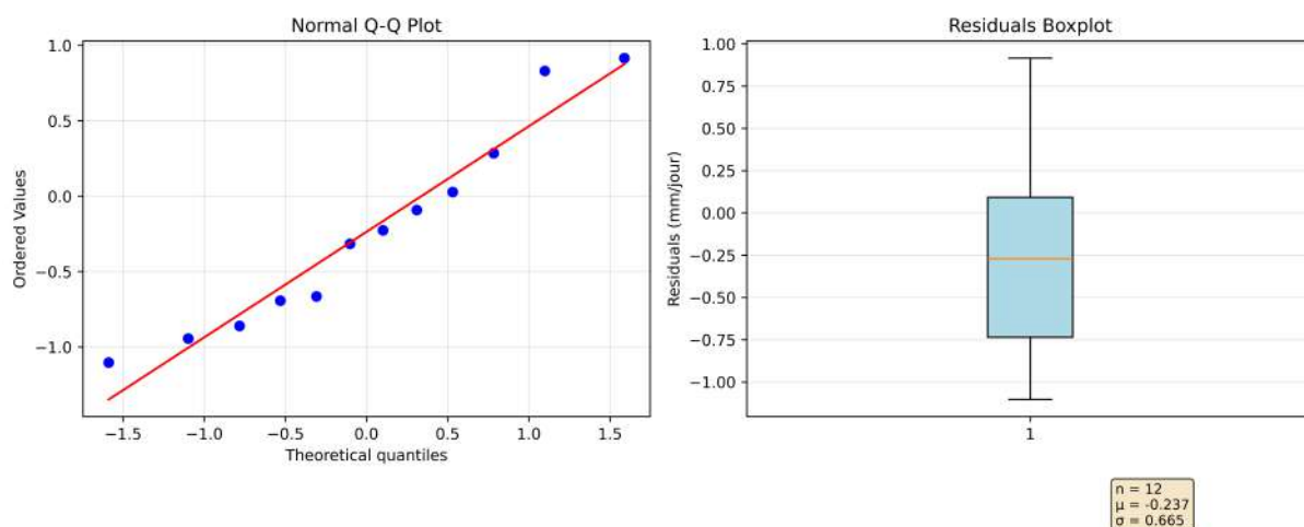
FIG. 4.17 : Tracé du Q-Q Plot et du boxplot des résidus confirmant la normalité.
