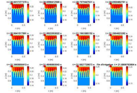
FIG. 4.11 : Évolution spatio-temporelle de la teneur en eau et progression du front d'irrigation jusqu'à la fin de l'irrigation pour la culture du maïs dans un sol sableux avec des données Open Meteo pour une localisation définie par 7.4 (latitude) ; 2.09 (longitude).
