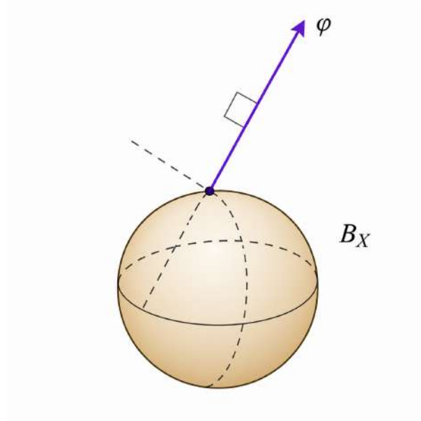
FIG. 2.4 : Espace de dualité
