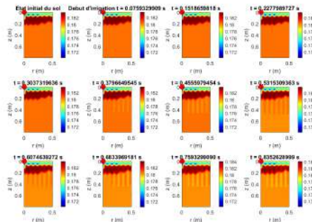
FIG. 4.12 : Évolution spatio-temporelle de la teneur en eau et progression du front au début de l'irrigation pour la culture de la tomate dans un sol sableux avec des données Open Meteo pour une localisation définie par 6.4 (latitude) ; 2.09 (longitude).
