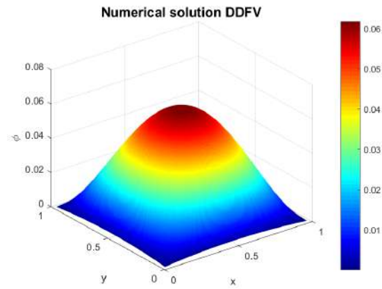
FIG. 2.9 : Solution numérique pour h = 0.04
