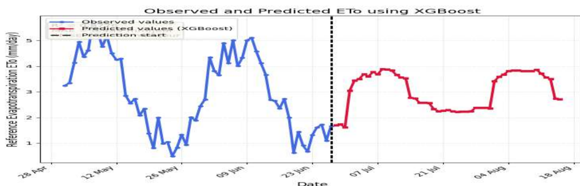
FIG. 4.18 : Prédiction de l'évapotranspiration avec XGBoost (eXtreme Gradient Boosting).
