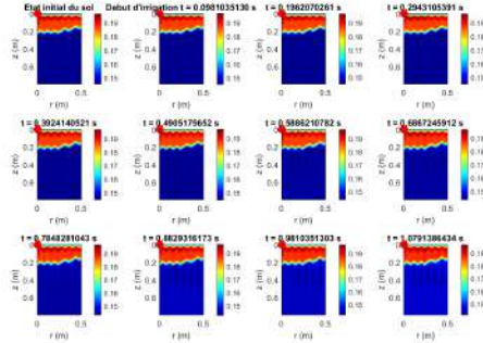
FIG. 4.10 : Évolution spatio-temporelle de la teneur en eau et progression du front d'irrigation au début de l'irrigation pour la culture du maïs dans un sol sableux avec des données Open Meteo pour une localisation définie par 7.4 (latitude) ; 2.09 (longitude).
