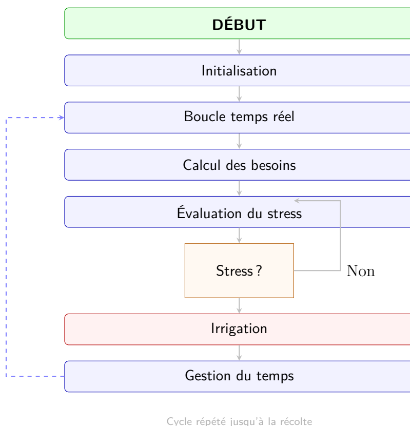
FIG. 3.4 : Algorithme du jumeau numérique descriptif (système d'irrigation en temps réel)
