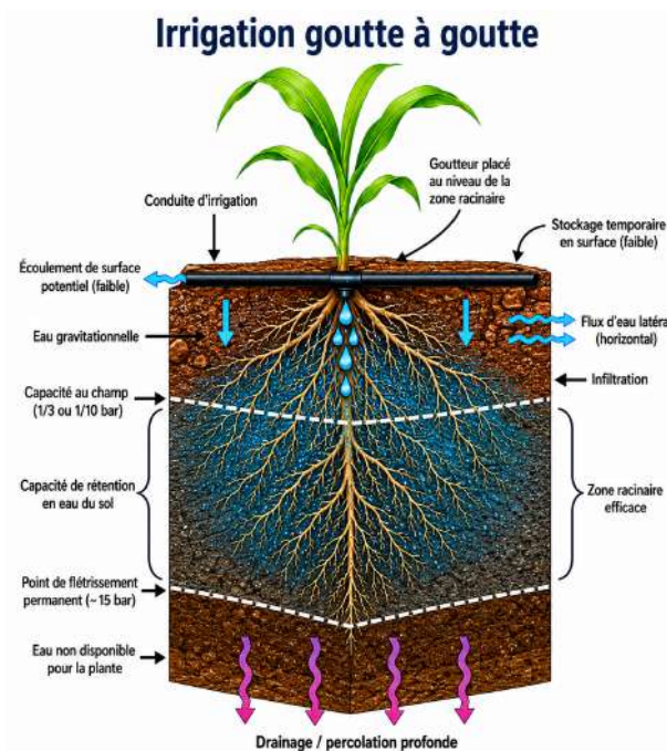
FIG. 1.4 : Schéma illustrant le fonctionnement de l'irrigation goutte à goutte. L'eau est appliquée localement au niveau de la zone racinaire par un goutteur, puis se déplace dans le sol par infiltration verticale et flux latéraux. La zone humidifiée constitue le réservoir d'eau disponible pour la plante entre la capacité au champ et le point de flétrissement permanent, tandis que l'excès d'eau est évacué par drainage profond.
