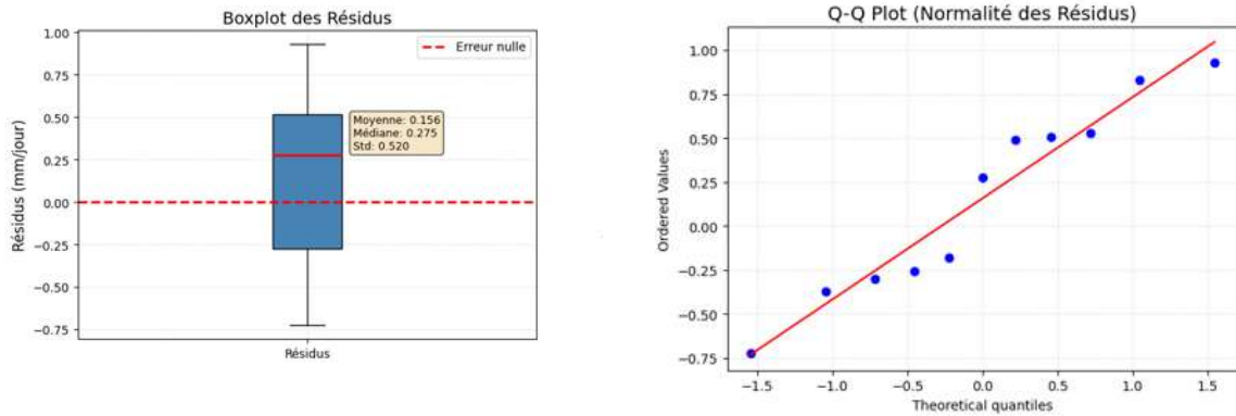
FIG. 4.19 : Tracé du Q-Q Plot et du boxplot des résidus confirmant la normalité.
