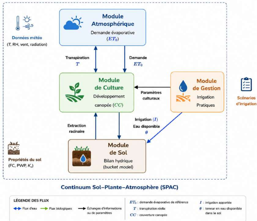
FIG. 1.15 : Architecture modulaire d'AquaCrop. Le modèle s'articule autour de quatre modules interconnectés qui simulent les interactions au sein du continuum sol-plante-atmosphère. Le module atmosphérique génère la demande évaporative, le module de culture calcule le développement de la canopée et la transpiration, le module de sol gère le bilan hydrique, et le module de gestion permet de définir les pratiques culturales.
