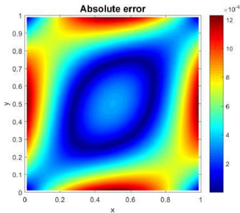
FIG. 2.15 : Erreur pour h = 0.02
