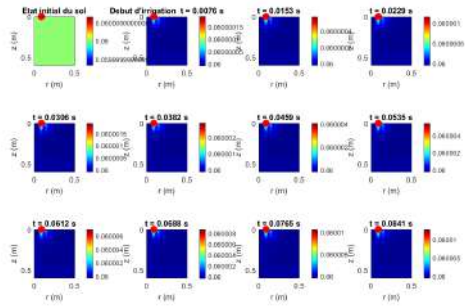
FIG. 4.5 : Évolution spatio-temporelle de la teneur en eau et progression du front au début de l'irrigation pour la culture du coton dans un sol sableux.
