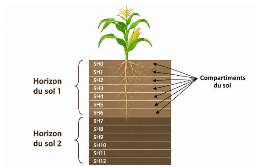
FIG. 3.5 : Horizons du sol, caractérisés par des paramètres physiques spécifiques du sol, et compartiments du sol introduits pour simuler la rétention, le mouvement de l'eau et des sels dans le profil du sol.
