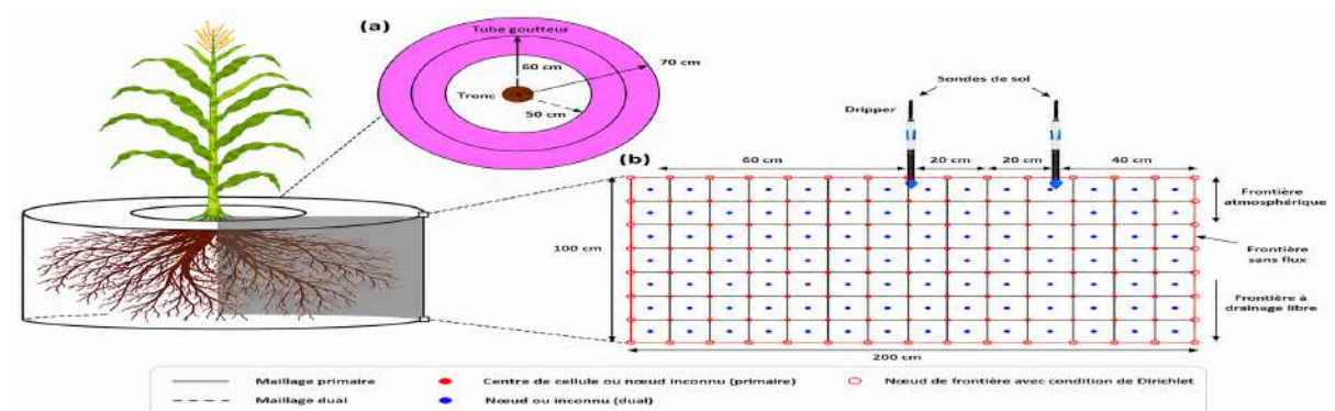
FIGURE 2.14 – Configuration du domaine de simulation pour l'irrigation goutte-à-goutte : géométrie axisymétrique, conditions aux limites et maillage primal-dual.
