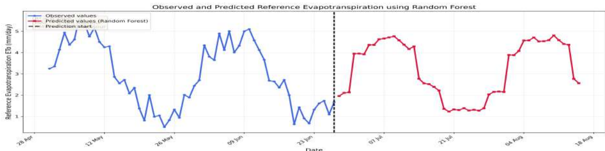
FIGURE 4.35 – Prédiction de l'évapotranspiration avec le Random Forest Regressor du moteur Data-Driven.
