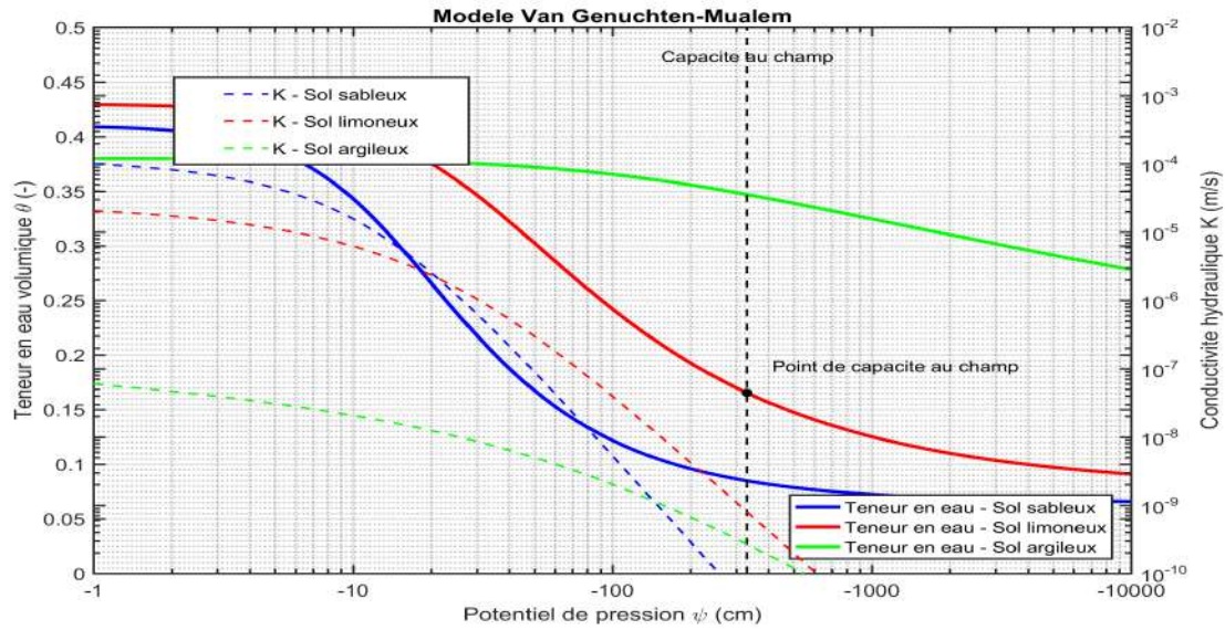
FIGURE 1.18 – Propriétés hydrauliques non linéaires de trois sols contrastés, représentées par les courbes de rétention de l'eau (SWRC) et les fonctions de conductivité hydraulique (HCF) selon le modèle de Van Genuchten-Mualem.
