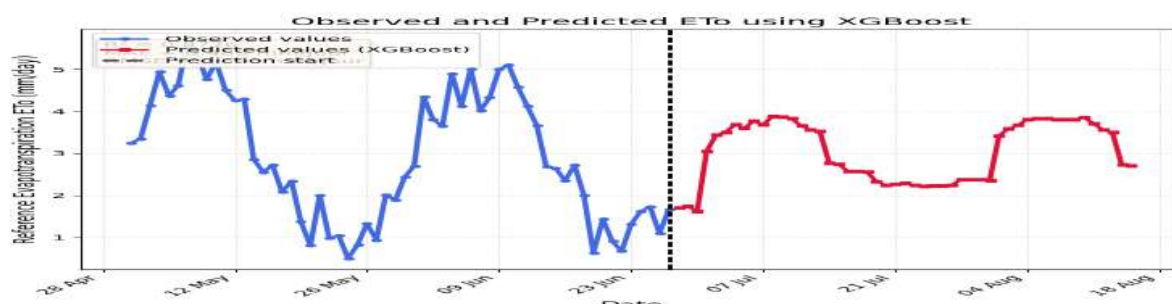
FIGURE 4.38 – Prédiction de l'évapotranspiration avec XGBoost (eXtreme Gradient Boosting).
