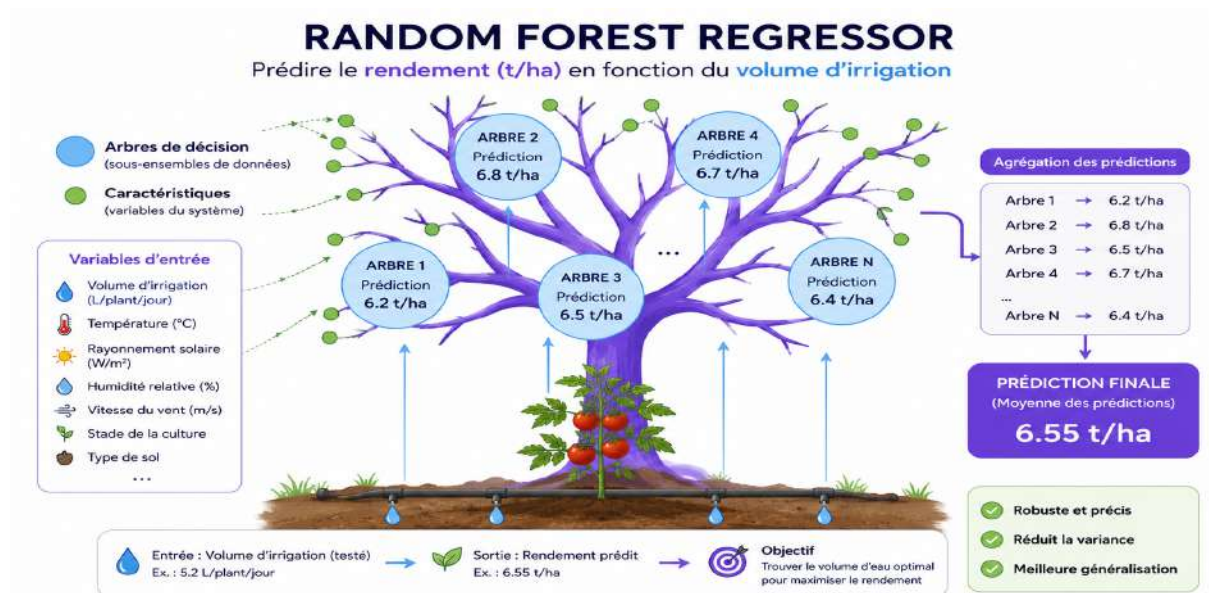
FIGURE 2.19 – Arbres de décision du Random Forest Regressor
