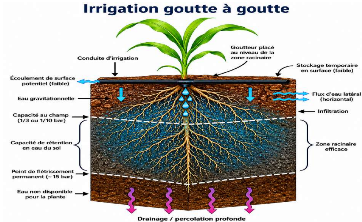
FIGURE 1.4 – Schéma illustrant le fonctionnement de l'irrigation goutte à goutte.
