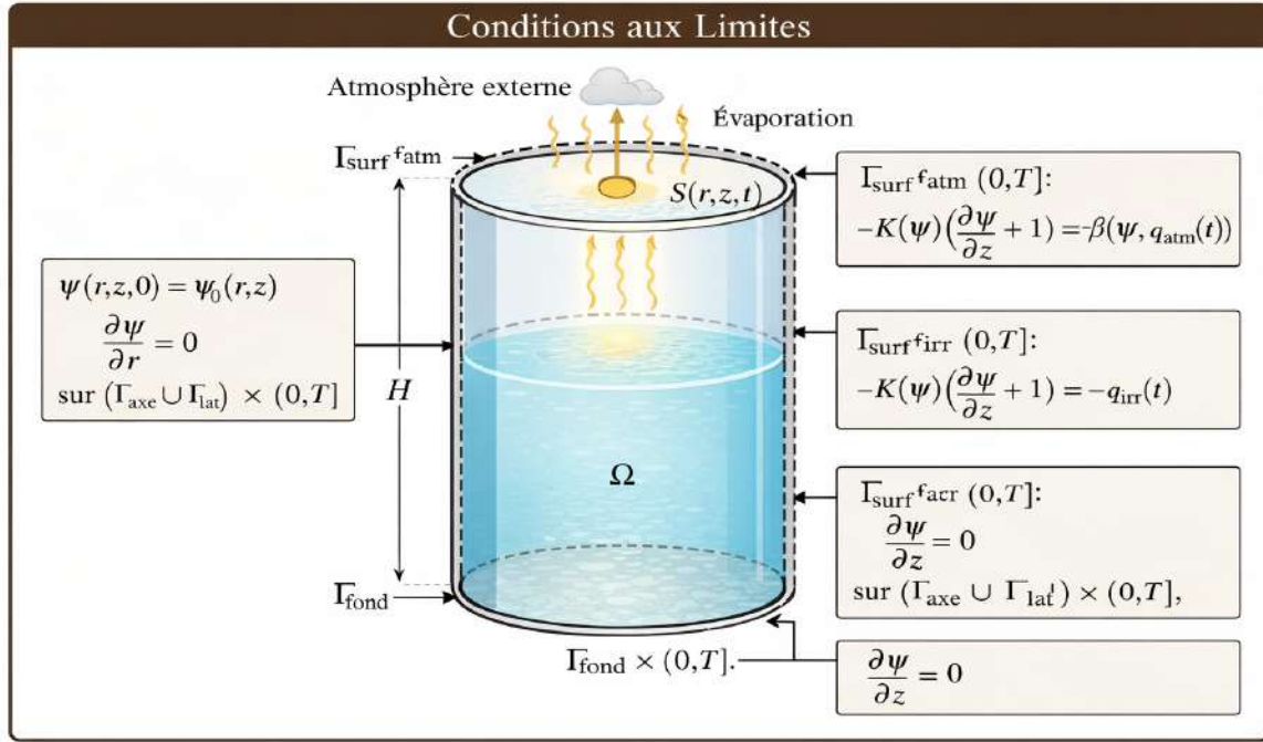
FIGURE 2.1 – Domaine de calcul et conditions aux limites en coordonnées cylindriques pour la simulation de l'irrigation goutte-à-goutte en géométrie 2D axisymétrique.
