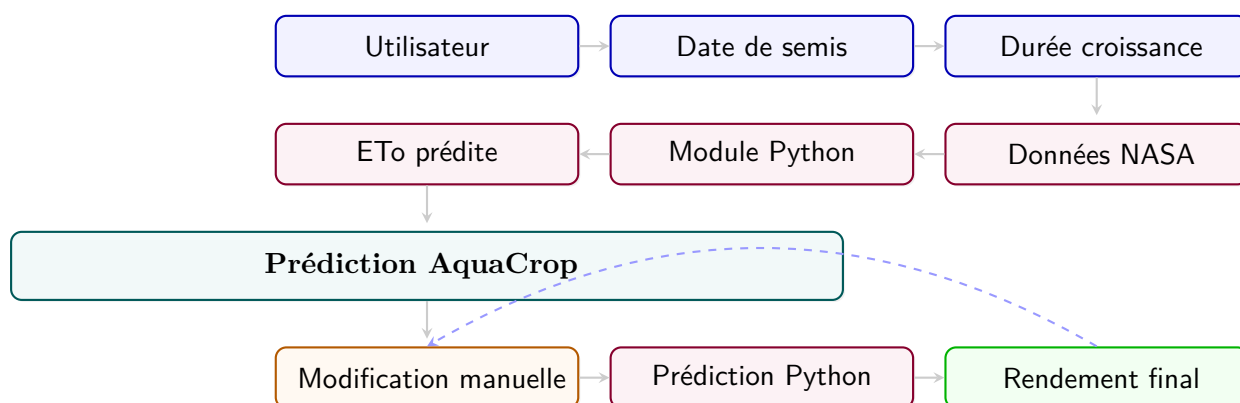
FIGURE 2.21 – Algorithme de prédiction du rendement par exploration de scénarios
