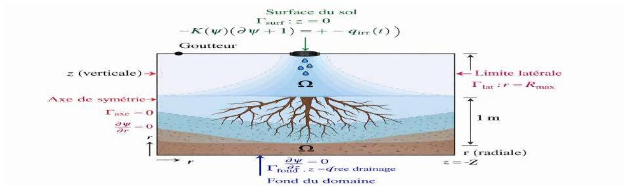
FIGURE 1.19 – Domaine de simulation axisymétrique et conditions aux limites appliquées à l'équation de Richards pour l'irrigation goutte-à-goutte.
