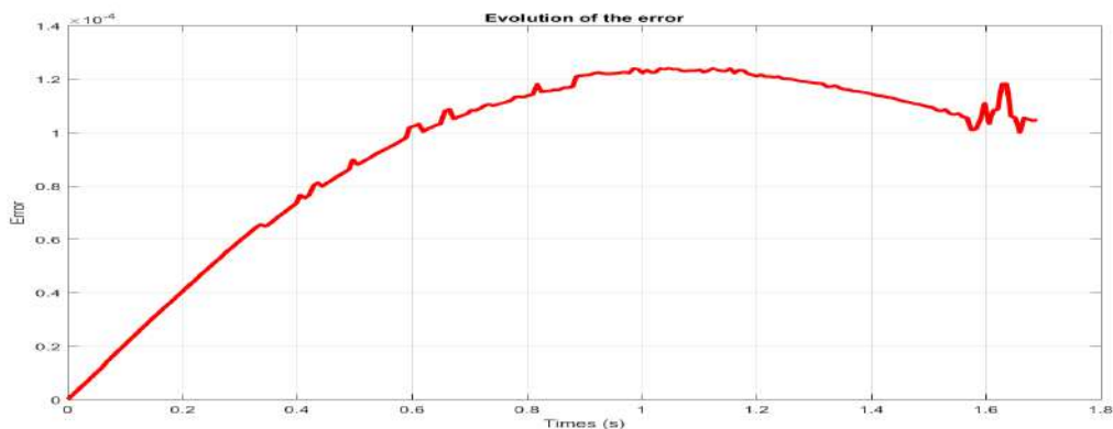
FIGURE 4.8 – Évolution de l'erreur pour la méthode d'itération de Picard.
