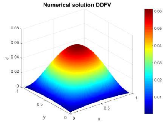
FIGURE 2.5 – Solution numérique pour h = 0,05
