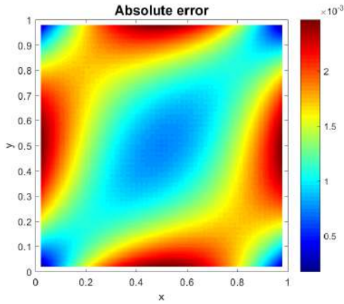
FIGURE 2.10 – Erreur pour h = 0,05
