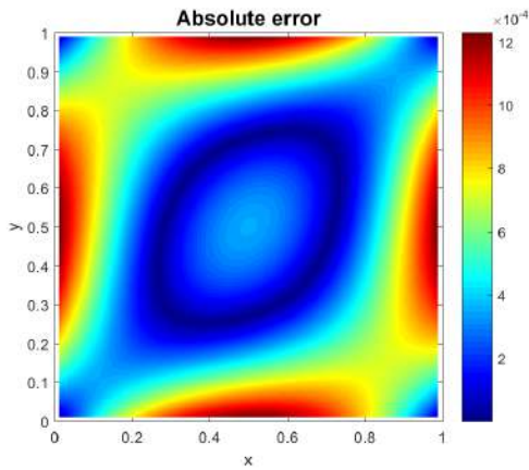
FIGURE 2.12 – Erreur pour h = 0,02
