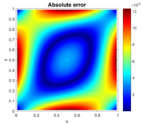
FIGURE 2.13 – Erreur pour h = 0,01
