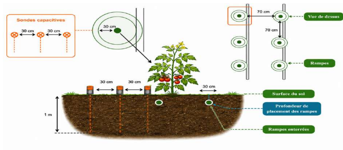
FIGURE 1.2 – Montage expérimental pour l'installation d'une rampe d'irrigation et de sondes capacitatives
