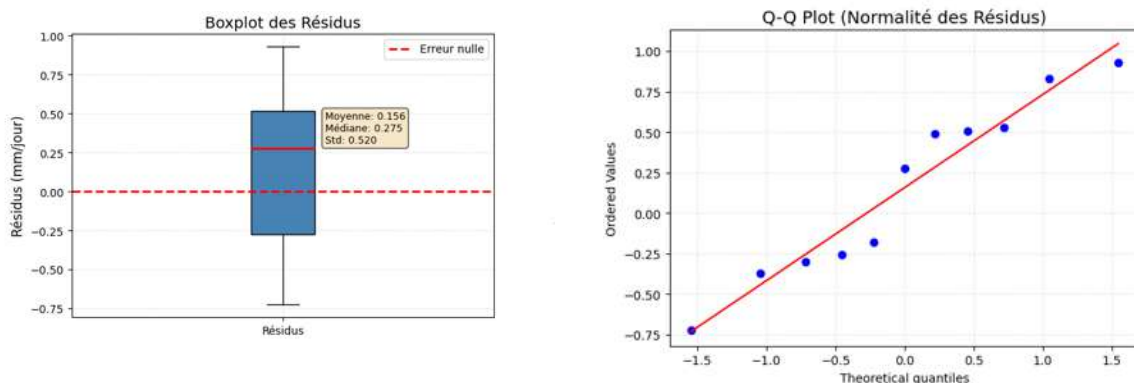
FIGURE 4.39 – Tracé du Q-Q Plot et du boxplot des résidus confirmant la normalité.
