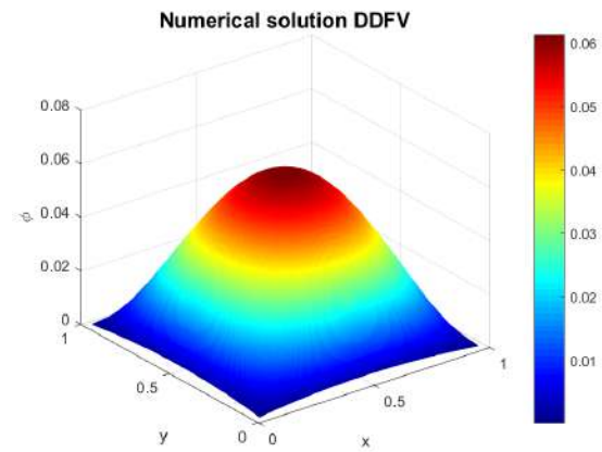
FIGURE 2.7 – Solution numérique pour h = 0,02
