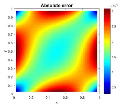
FIGURE 2.9 – Erreur pour h = 0,1
