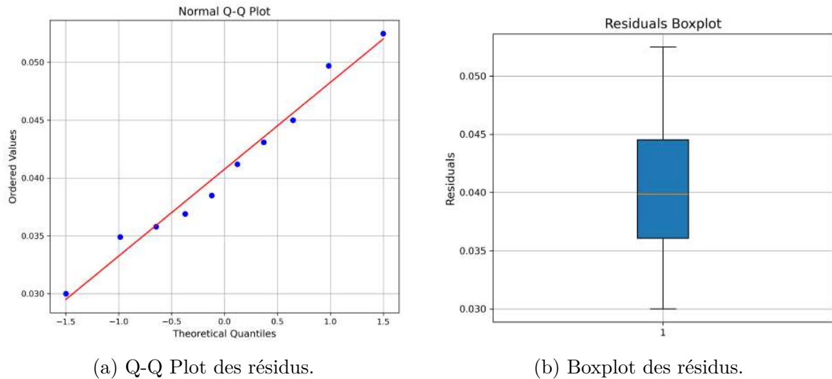
FIGURE 4.9 – Q-Q Plot et boxplot des résidus confirmant la normalité.
