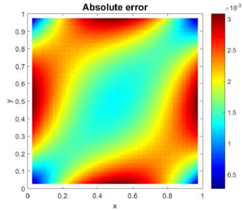
FIGURE 2.11 – Erreur pour h = 0,04
