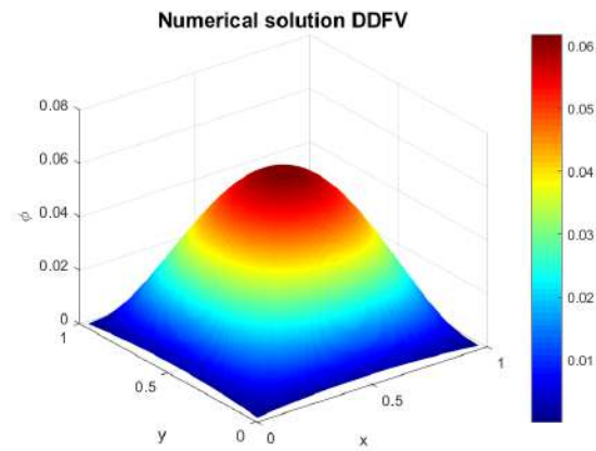
FIGURE 2.6 – Solution numérique pour h = 0,04
