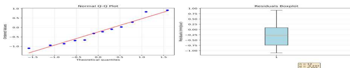
FIGURE 4.37 – Tracé du Q-Q Plot et du boxplot des résidus confirmant la normalité.
