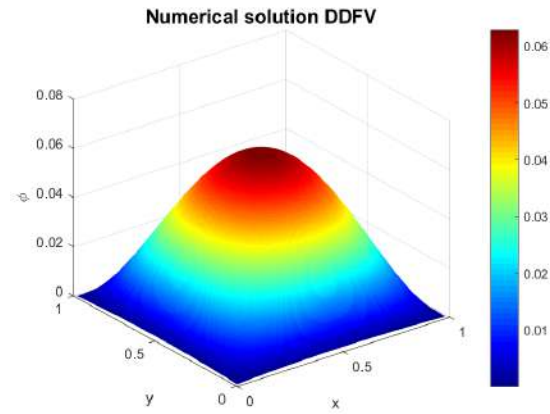
FIGURE 2.4 – Solution numérique pour h = 0,1
