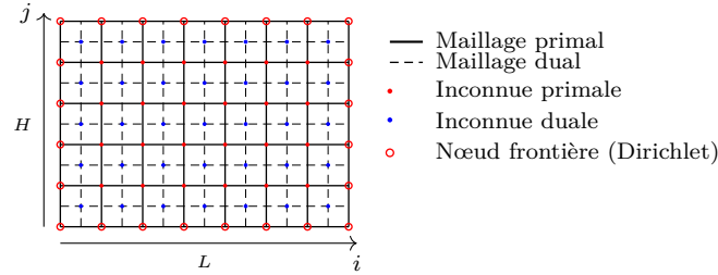
FIGURE 2.2 – Maillage volumes finis en dualité discrète.
