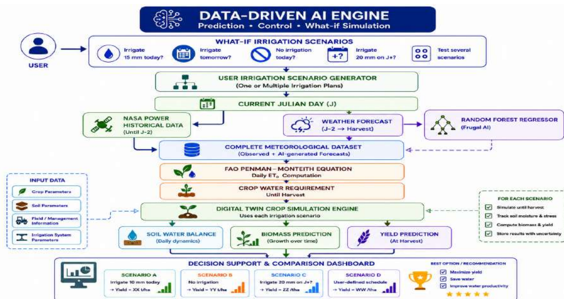
FIGURE 2.17 – Fonctionnement du moteur Data-Driven AI.
