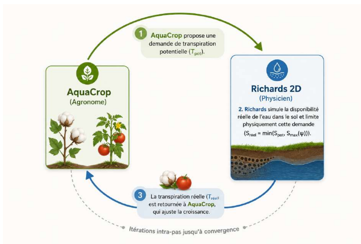
FIGURE 2.15 – Schéma du couplage bidirectionnel fort entre AquaCrop et le solveur Richards.
