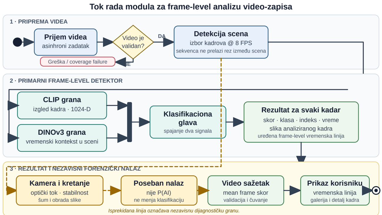
UML dijagram. Tok rada modula za frame-level analizu video-zapisa
