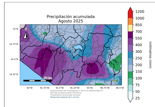
(b) Precipitación acumulada para el mes de agosto de 2025 dado por el registro de datos ENACTS.
