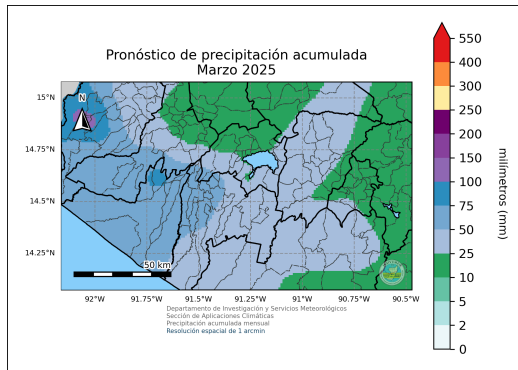
(a) Pronóstico de precipitación acumulada para el mes de marzo de 2025 dado por la LSTM.
