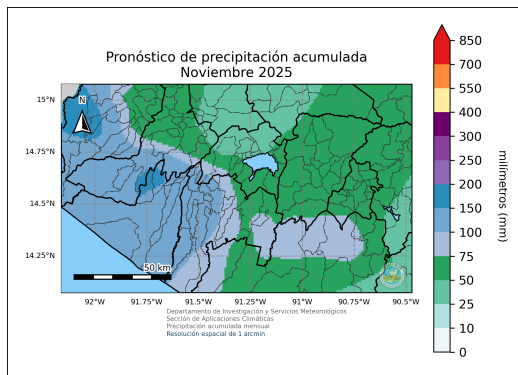
(a) Pronóstico de precipitación acumulada para el mes de noviembre de 2025 dado por la LSTM.
