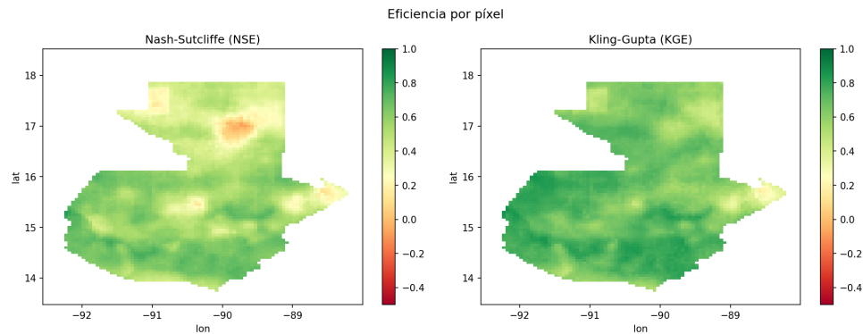
Fig. 5.3: NSE y KGE para el territorio nacional en los datos de validación del entrenamiento.
