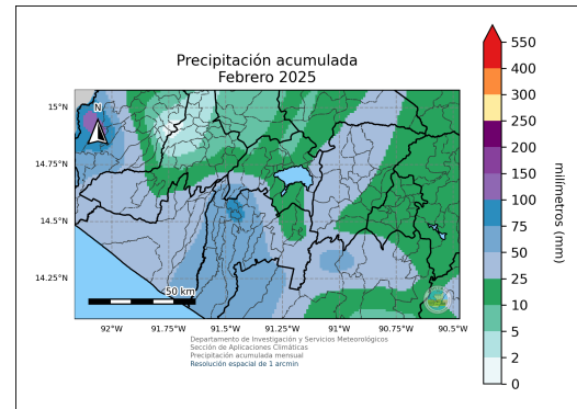
(b) Precipitación acumulada para el mes de febrero de 2025 dado por el registro de datos ENACTS.
