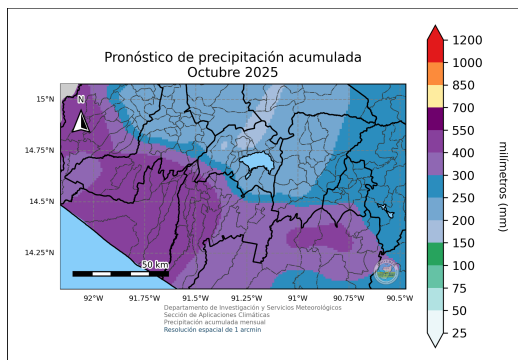
(a) Pronóstico de precipitación acumulada para el mes de octubre de 2025 dado por la LSTM.
