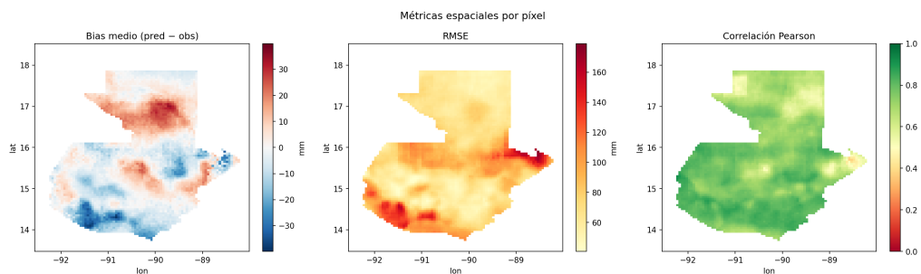
Fig. 5.4: Sesgo medio, RMSE y correlación de Pearson para el territorio nacional en los datos de validación del entrenamiento.
