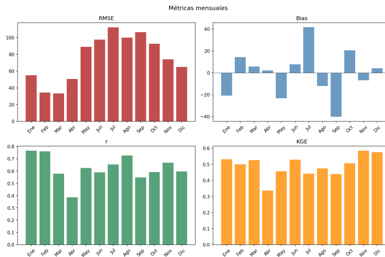
Fig. 5.5: RMSE, sesgo medio, correlación de Pearson y coeficiente de Kling-Gupta mensuales medios para los datos de validación del entrenamiento.
