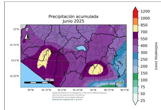
(b) Precipitación acumulada para el mes de junio de 2025 dado por el registro de datos ENACTS.
