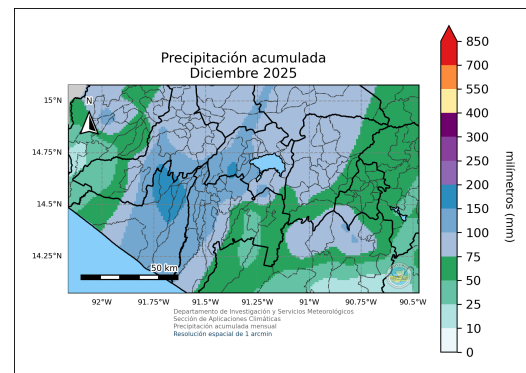
(b) Precipitación acumulada para el mes de diciembre de 2025 dado por el registro de datos ENACTS.
