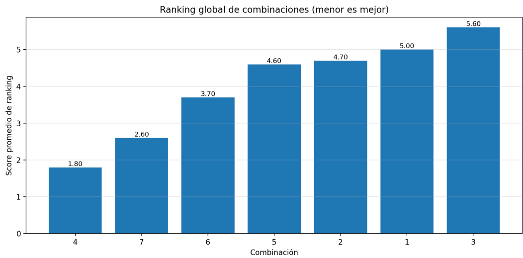
Fig. 5.2: Los resultados muestran que la combinación óptima de predictores fue: SST, tp y MJO.
