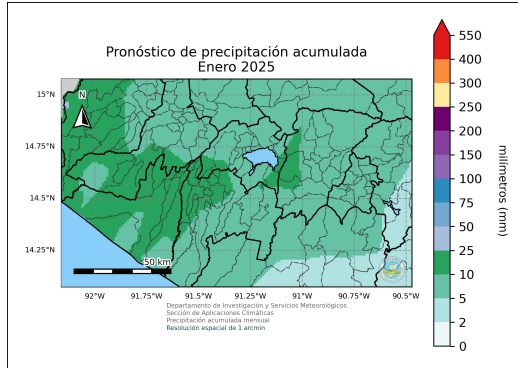
(a) Pronóstico de precipitación acumulada para el mes de enero de 2025 dado por la LSTM.
