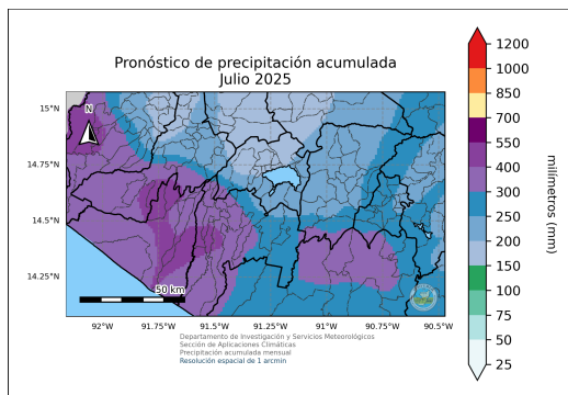
(a) Pronóstico de precipitación acumulada para el mes de julio de 2025 dado por la LSTM.
