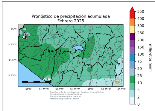
(a) Pronóstico de precipitación acumulada para el mes de febrero de 2025 dado por la LSTM.
