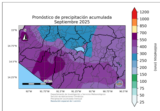
(a) Pronóstico de precipitación acumulada para el mes de septiembre de 2025 dado por la LSTM.
