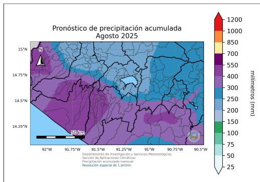
(a) Pronóstico de precipitación acumulada para el mes de agosto de 2025 dado por la LSTM.
