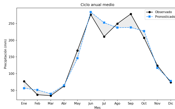
Fig. 5.6: Precipitación media mensual para los datos de validación del entrenamiento en el territorio nacional.
