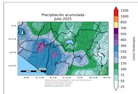
(b) Precipitación acumulada para el mes de julio de 2025 dado por el registro de datos ENACTS.
