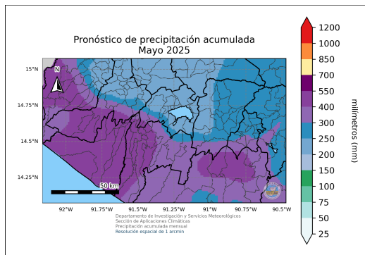
(a) Pronóstico de precipitación acumulada para el mes de mayo de 2025 dado por la LSTM.
