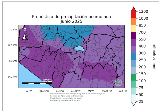
(a) Pronóstico de precipitación acumulada para el mes de junio de 2025 dado por la LSTM.
