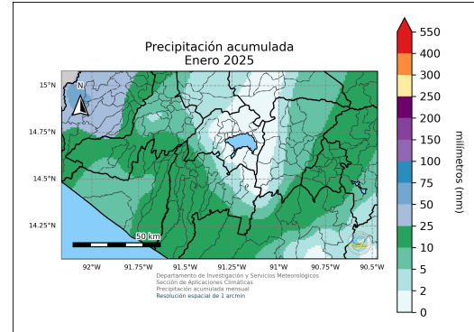
(b) Precipitación acumulada para el mes de enero de 2025 dado por el registro de datos ENACTS.
