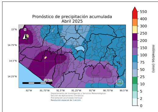
(a) Pronóstico de precipitación acumulada para el mes de abril de 2025 dado por la LSTM.
