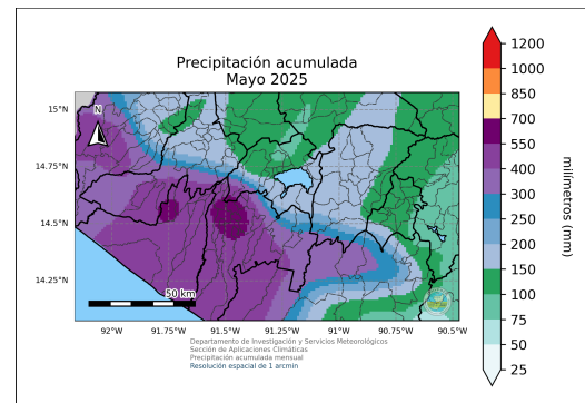
(b) Precipitación acumulada para el mes de mayo de 2025 dado por el registro de datos ENACTS.
