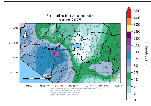
(b) Precipitación acumulada para el mes de marzo de 2025 dado por el registro de datos ENACTS.
