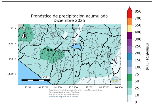
(a) Pronóstico de precipitación acumulada para el mes de diciembre de 2025 dado por la LSTM.
