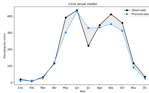
Fig. 5.8: Precipitación media mensual para los datos de validación del entrenamiento en la región de Bocacosta.
