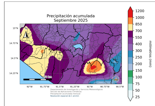
(b) Precipitación acumulada para el mes de septiembre de 2025 dado por el registro de datos ENACTS.
