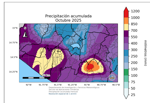
(b) Precipitación acumulada para el mes de octubre de 2025 dado por el registro de datos ENACTS.
