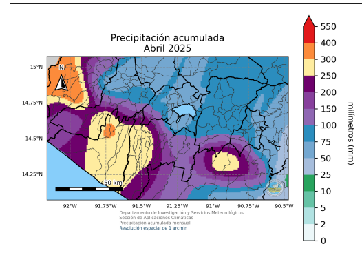
(b) Precipitación acumulada para el mes de abril de 2025 dado por el registro de datos ENACTS.
