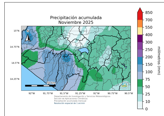
(b) Precipitación acumulada para el mes de noviembre de 2025 dado por el registro de datos ENACTS.
