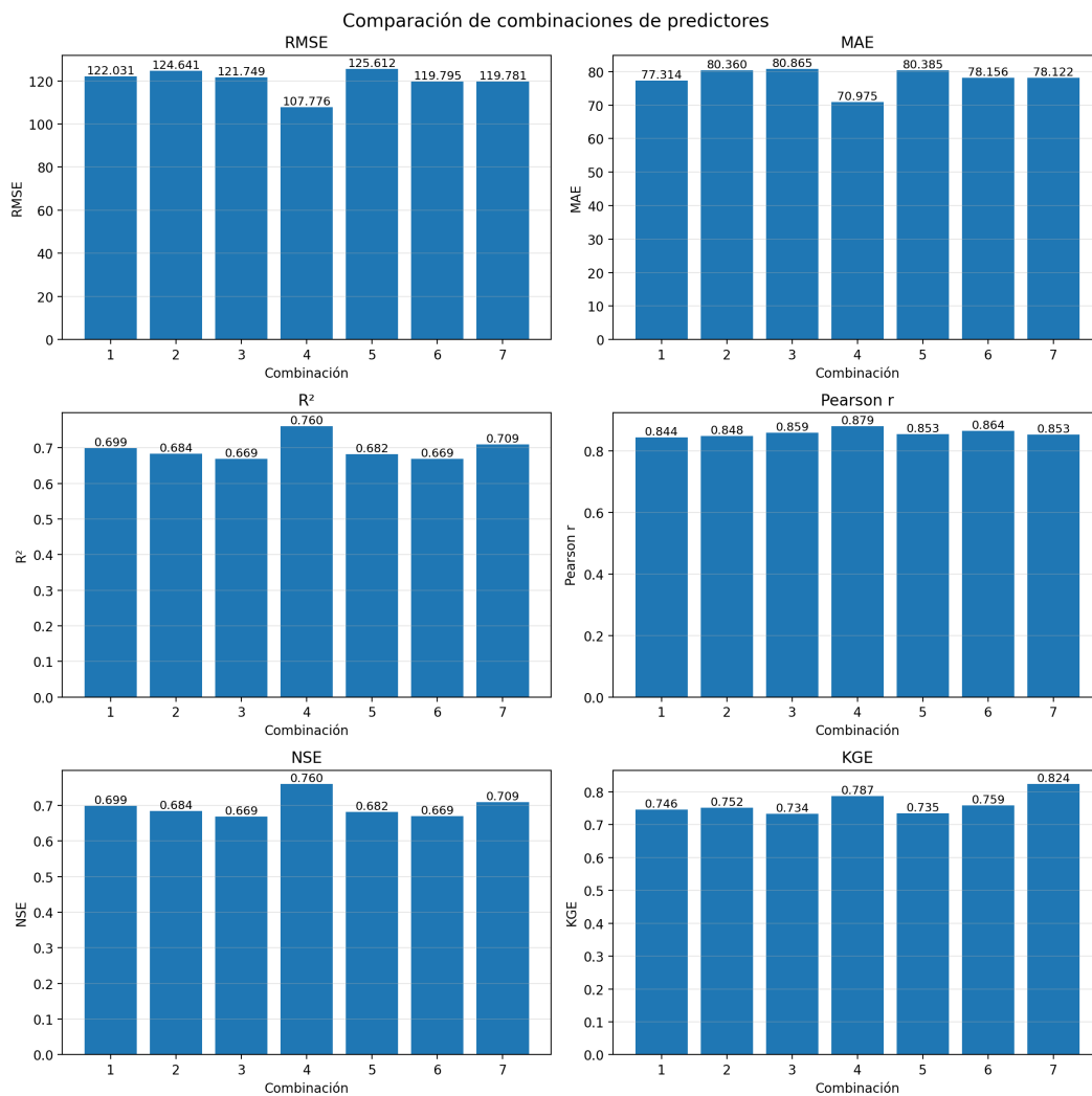
Fig. 5.1: Comparación de métricas para distintos predictores
