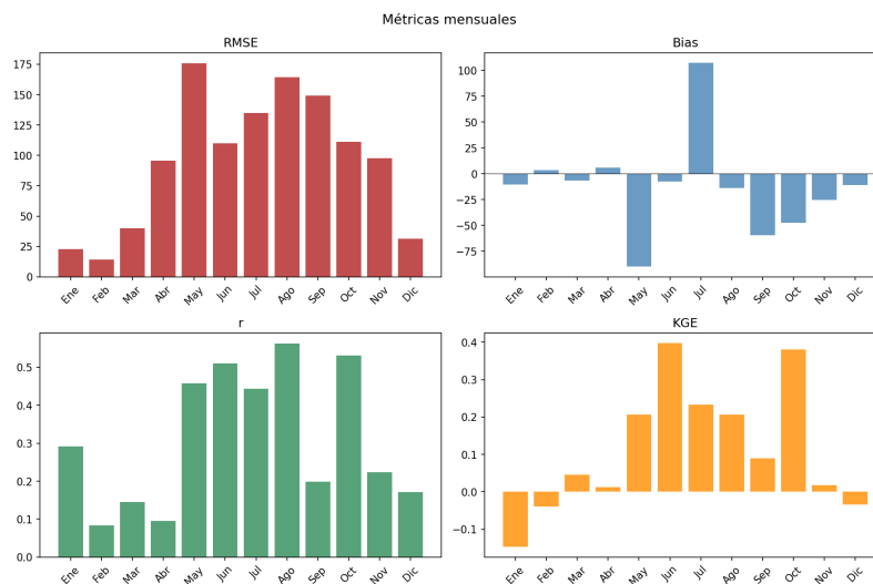
Fig. 5.7: RMSE, sesgo medio, correlación de Pearson y coeficiente de Kling-Gupta mensuales medios para los datos de validación del entrenamiento en la región de Bocacosta.
