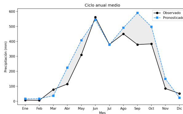
Fig. 5.15: Precipitación media mensual para los datos de validación del entrenamiento en la región de Bocacosta.
