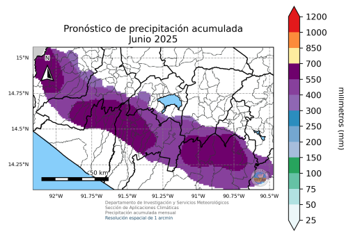
(a) Pronóstico de precipitación acumulada para el mes de junio de 2025 dado por la LSTM.
