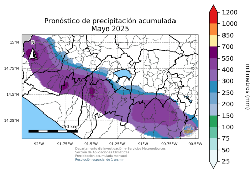
(a) Pronóstico de precipitación acumulada para el mes de mayo de 2025 dado por la LSTM.
