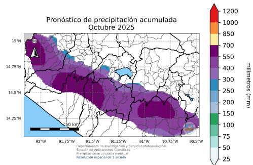
(a) Pronóstico de precipitación acumulada para el mes de octubre de 2025 dado por la LSTM.
