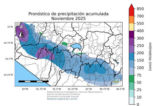
(a) Pronóstico de precipitación acumulada para el mes de noviembre de 2025 dado por la LSTM.
