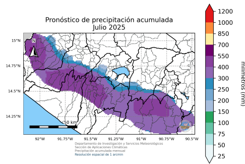
(a) Pronóstico de precipitación acumulada para el mes de julio de 2025 dado por la LSTM.
