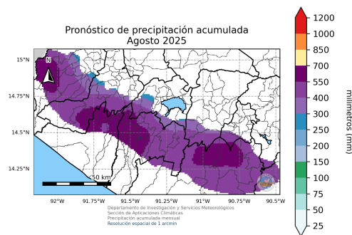
(a) Pronóstico de precipitación acumulada para el mes de agosto de 2025 dado por la LSTM.
