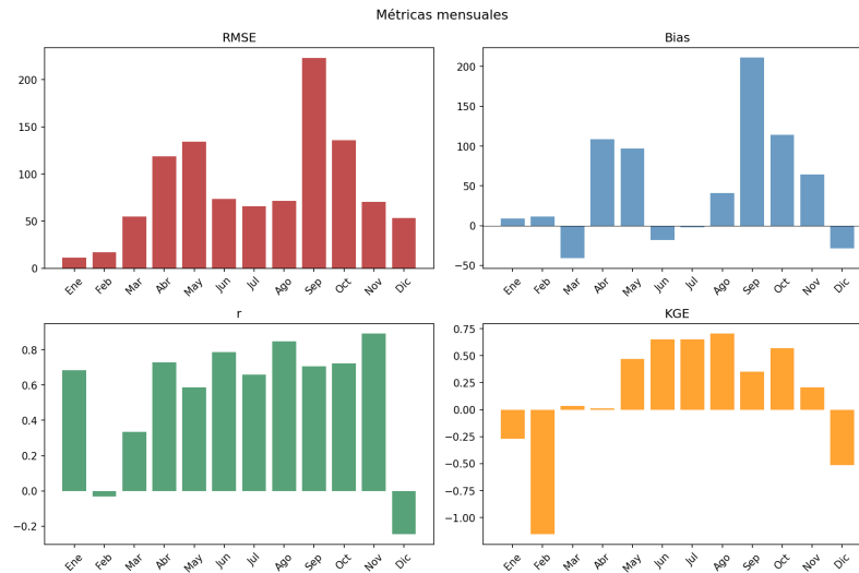
Fig. 5.14: RMSE, sesgo medio, correlación de Pearson y coeficiente de Kling-Gupta mensuales medios para los datos de validación del entrenamiento en la región de Bocacosta.
