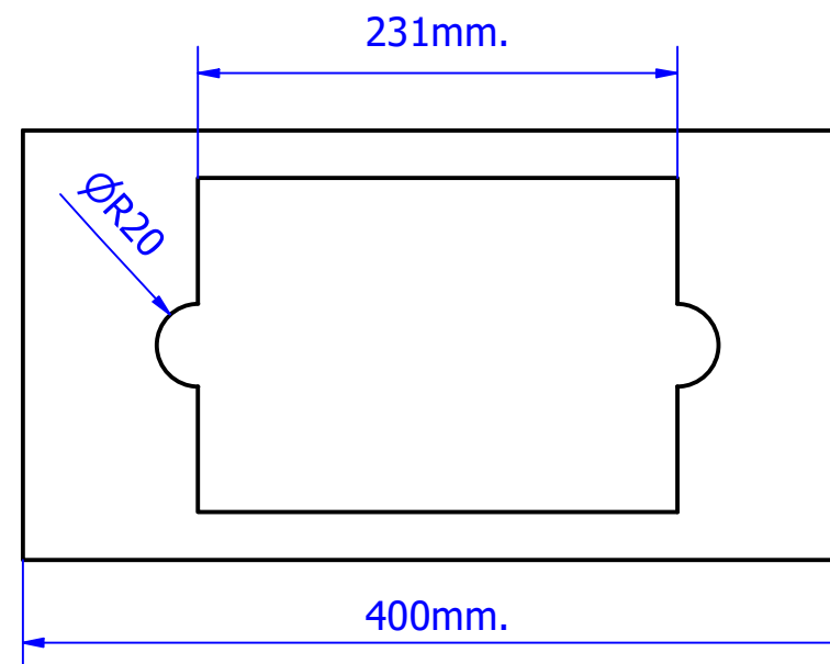
PIEZA N°5: BASE TERCER PISO (L. IZQ)
