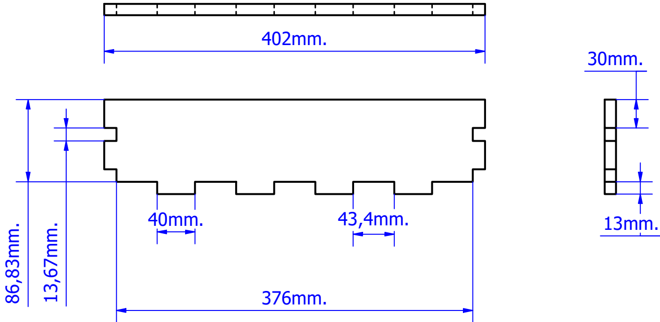
PIEZA N°8: PLACA VERTICAL INFERIOR 1ER PISO (L.IZQ.)
