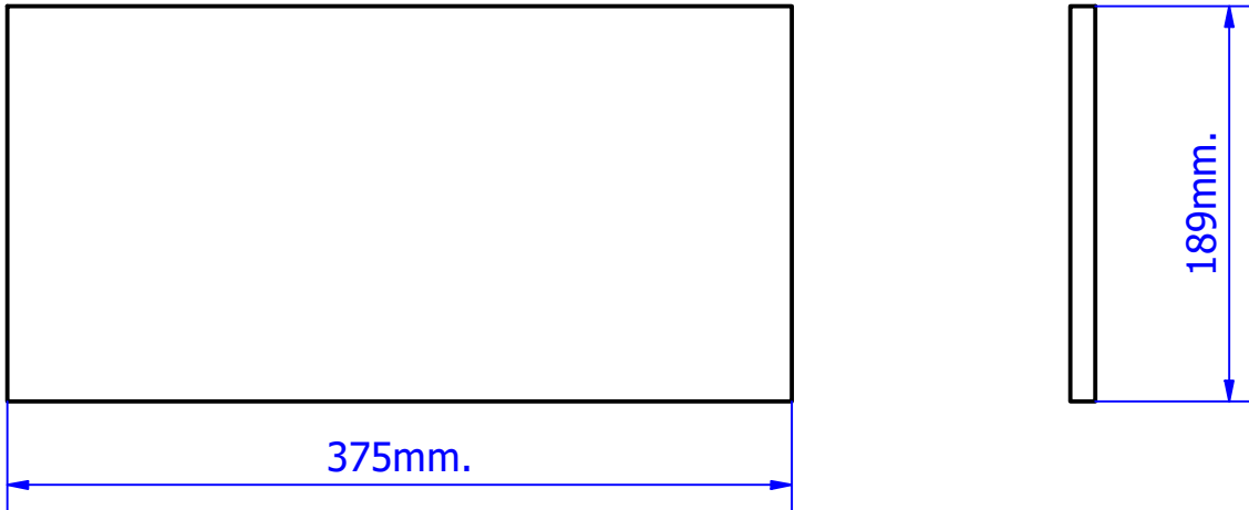
PIEZA N°9: PLACA MÓVIL 2DO PISO (L.IZQ)
