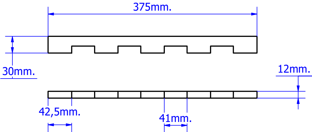
PIEZA N°6: PIEZA SUPERIOR DE ELEVACIÓN TRASERA (L. IZQ.)
