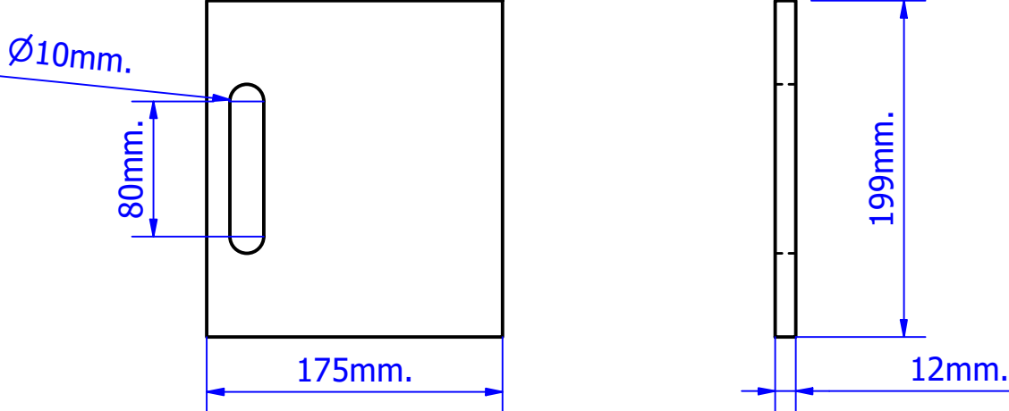
PIEZA N°24: PUERTA INTERNA (L.DRCH.)
