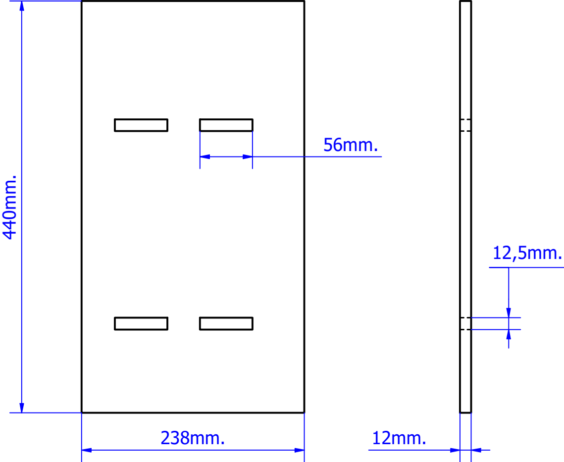
PIEZAS N°19 Y 20: PLACAS LATERALES (L.DRCH.)
