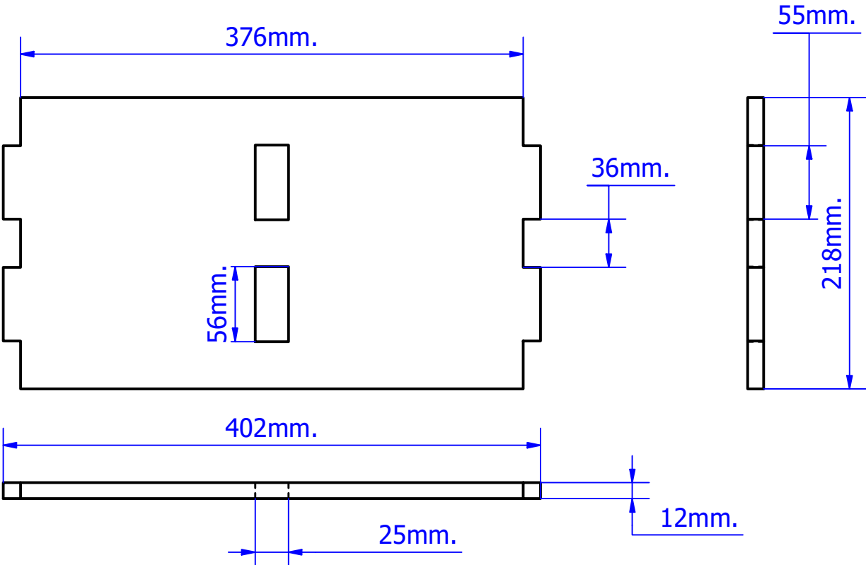
PIEZA N°24: PUERTA INTERNA (L.DRCH.)
