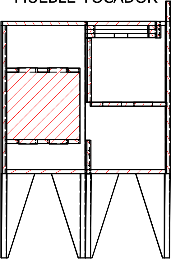
CORTE A-A ( 1 : 7 ) MUEBLE TOCADOR
