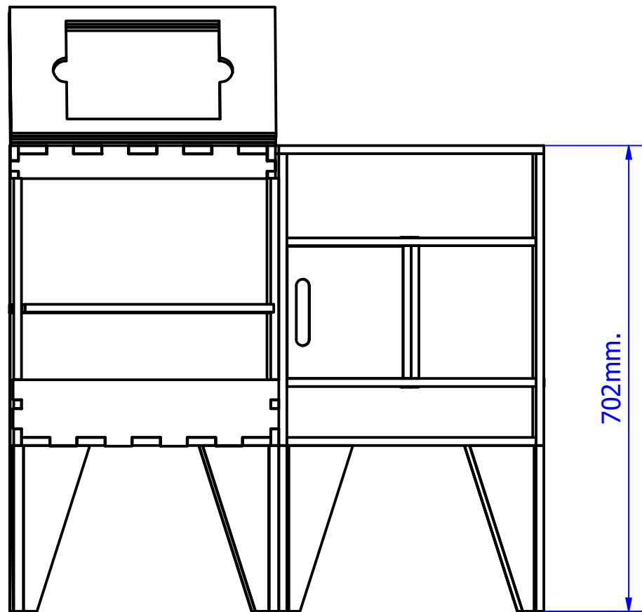
MUEBLE TOCADOR: VISTA FRONTAL
