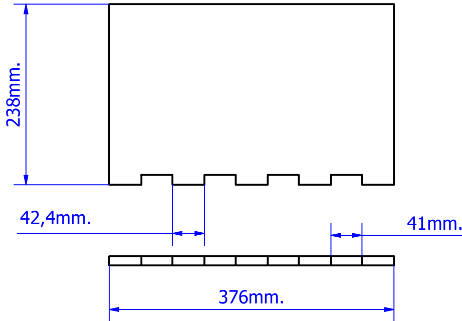
PIEZA N°13: PLACA INFERIOR GENERAL (L.IZQ.)
