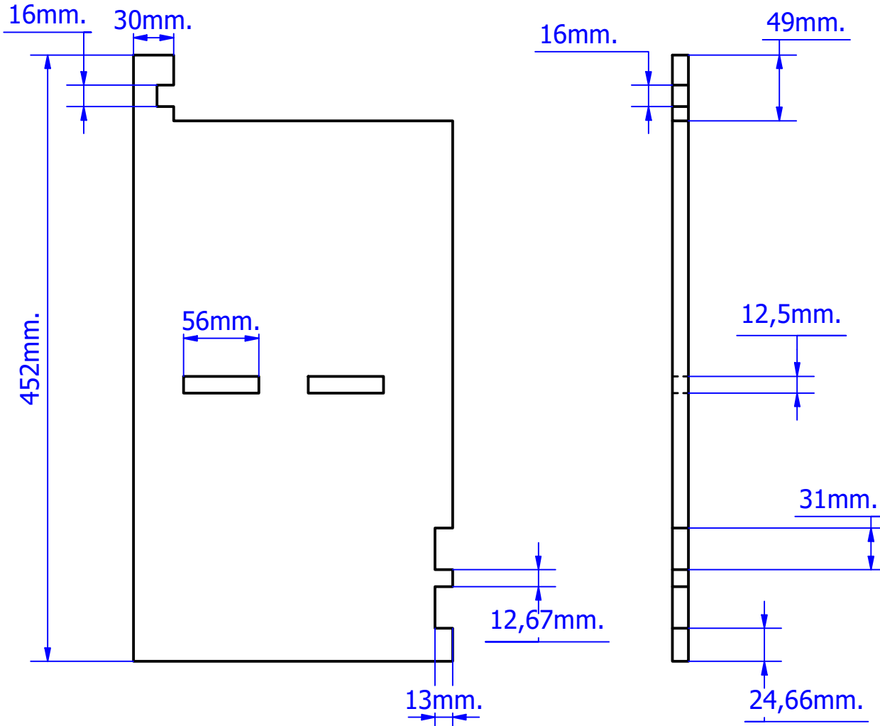
PIEZAS N°11 Y 12: PLACAS LATERALES PRINCIPALES (L.IZQ.)
