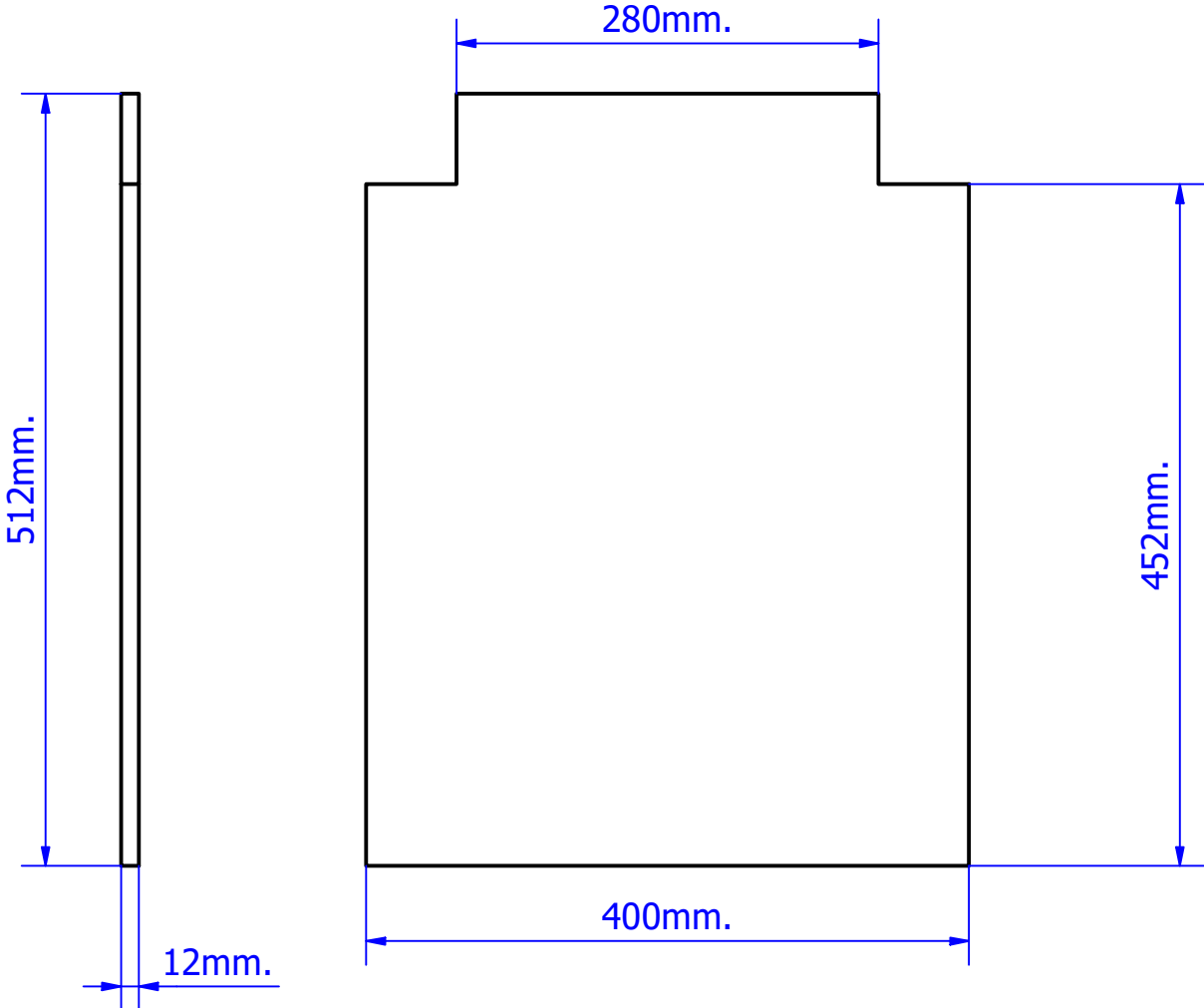
PIEZA N°13: PLACA INFERIOR GENERAL (L.IZQ.)
