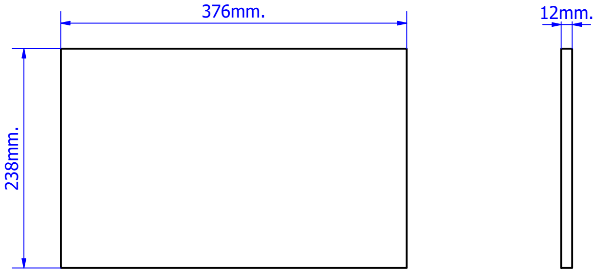
PIEZA N°14: PLACA BASE (L.DRCH.)
