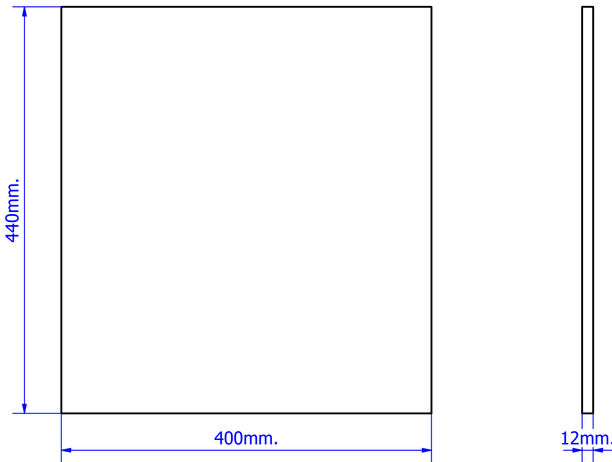
PIEZA N°15: PLACA TRASERA (L.DRCH.)
