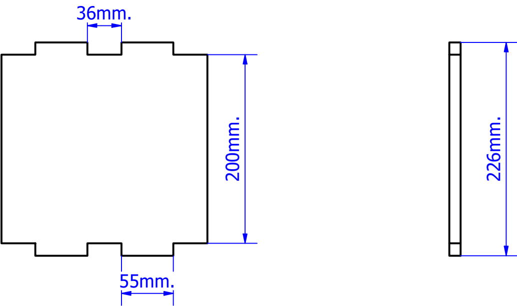
PIEZAS N° 16 Y 17: DIVISIONES 2DO PISO (L.DRCH.)
