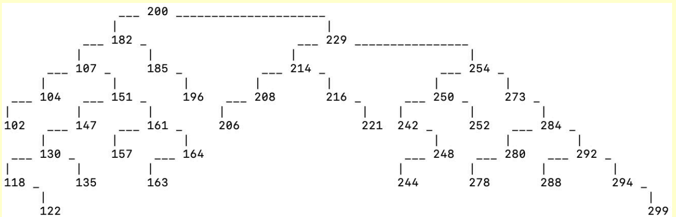
Árbol antes de eliminar el nodo 182
