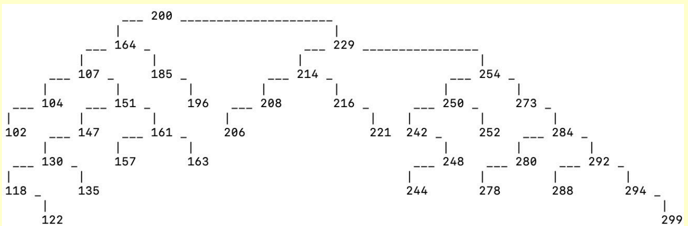
Árbol después de eliminar el nodo 182
