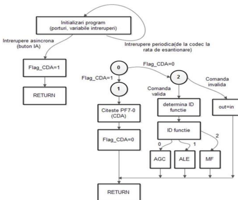
Inițializări program : Se configurează porturile (PF-urile ca intrări, Afișorul ca ieșire), se inițializează bufferele circulare de recepție și transmisie (rx_buf și tx_buf), începe activitatea CODEC și se activează întreruperile.
