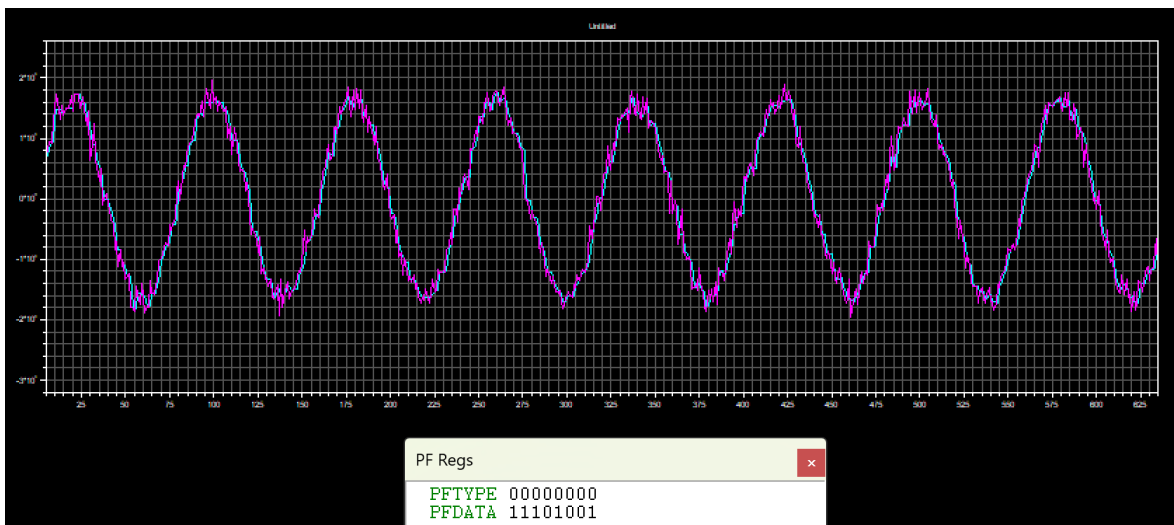
Semnal intrare&iesire canal dreapta
