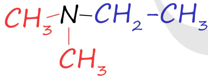
диметилэтиламин
