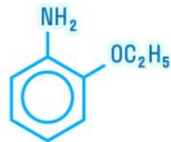
м-фенетидин
