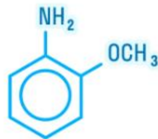
о-анизидин
