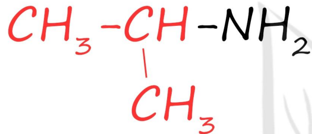
изопропиламин
