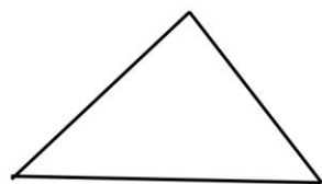
циклопропан
