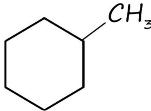
метилциклогексан
