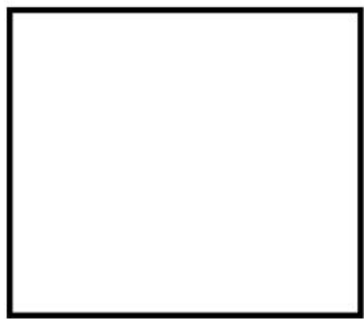
циклобутан
