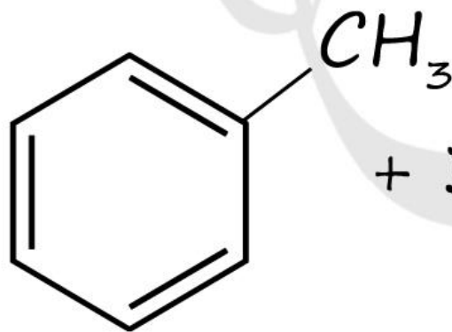
толуол
