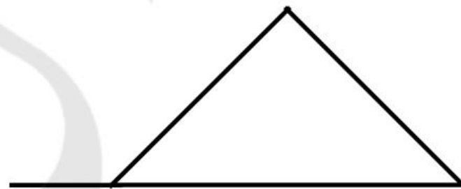
метилциклопропан
