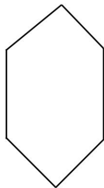
циклогексан
