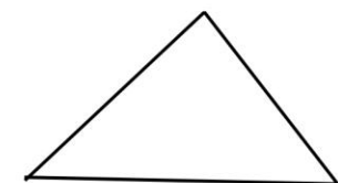
циклопропан
