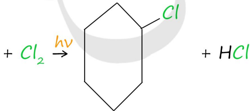
хлорциклогексан
