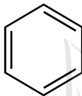
бензол
