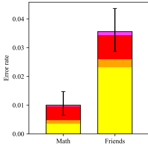
Grok 3 Mini Beta (high) – error types
