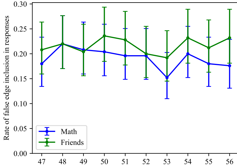
Grok 3 Mini Beta (high) – false edges
