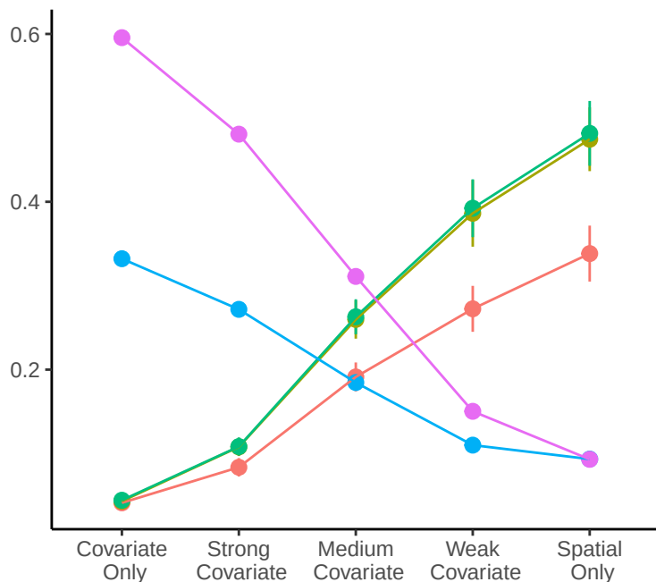
Interval Width
