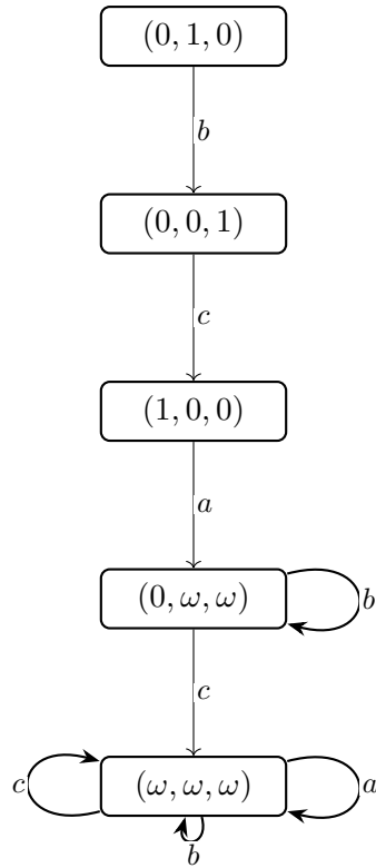
Abbildung 1: Überdeckungsgraph für das Petrinetz P_4
