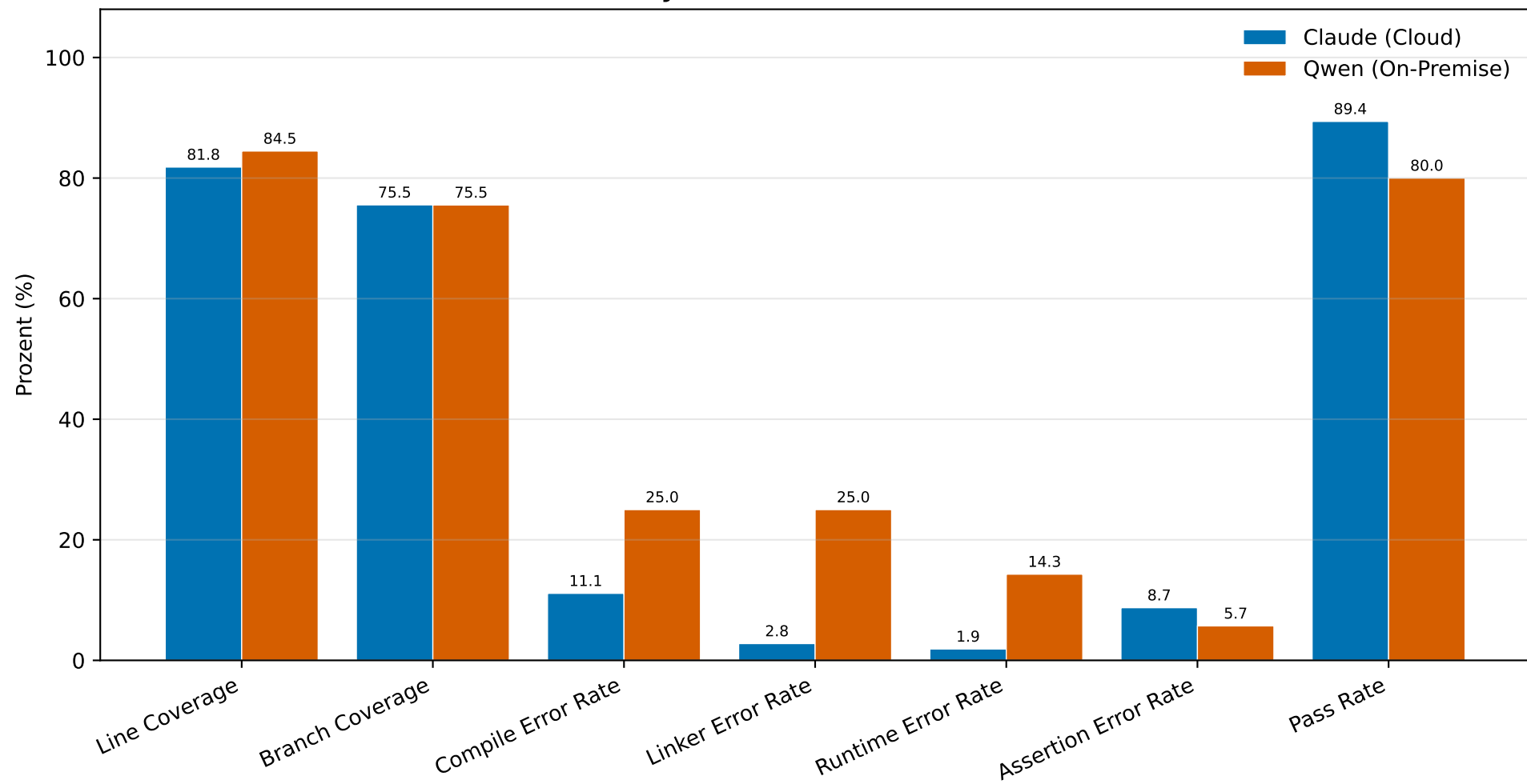
LLM-Performance je Metrik (Mittel ueber alle Codebases)
