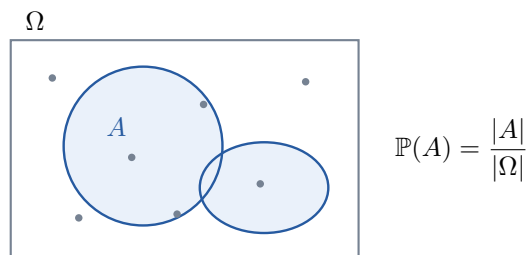
Фигура 1: Геометрична вероятност: вероятността на A е делът от площта на \Omega , който A заема. Броенето на изходи е безсмислено — те са неизброимо много и всеки поотделно има вероятност нула — но площта остава смислена мярка. Точката пада „наслуки“: равномерно върху \Omega , така че равни площи имат равни вероятности.
