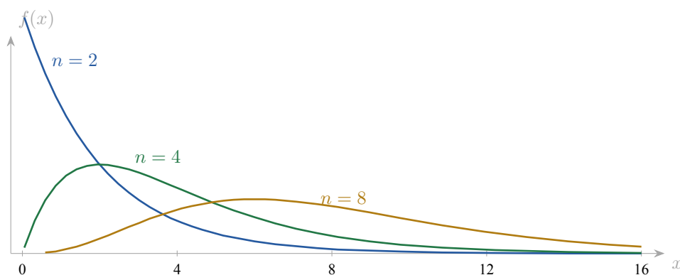
Фигура 9.2: Плътността на \chi^2(n) за три стойности на n . С растене на n върхът се измества надясно и кривата се сплесква — очакването е n , а дисперсията 2n . Разпределението живее само върху положителната полуос (то е сума от квадрати) и е силно несиметрично при малки n ; точно затова доверителният интервал за дисперсията в лекция 13 се нуждае от два различни квантила, а не от \pm q както при нормалното.
