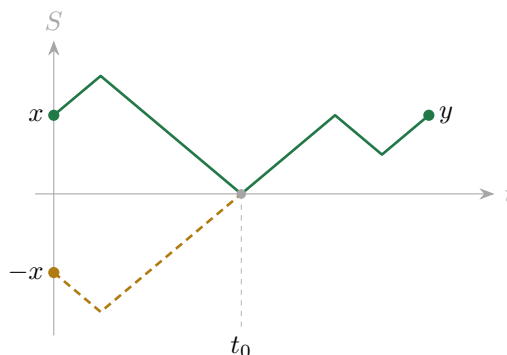
Фигура 15.1: Принциплът на отражението. Плътната линия е „лош“ път от (0, x) до (n, y) ; t_0 е първият момент, в който той докосва оста. Отразявайки началната част до момента t_0 спрямо оста (прекъснатата линия), получаваме път от (0, -x) до (n, y) . Съответствието е биекция.
