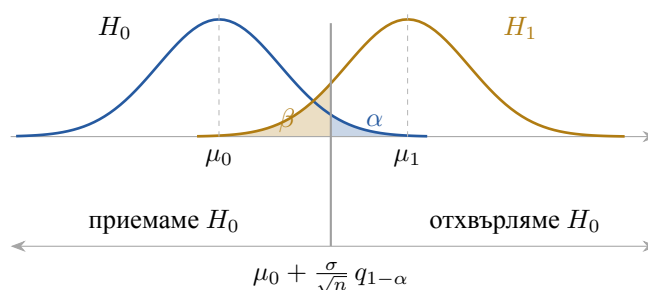
Фигура 13.2: Двете хипотези и решението между тях. Под H_0 средното е \mu_0 , под H_1 е \mu_1 > \mu_0 ; наблюденията се сравняват с прага \mu_0 + \frac{\sigma}{\sqrt{n}} q_{1-\alpha} . Вдясно от прага отхвърляме H_0 . Заштрихованата площ под лявата крива е \alpha — вероятността да отхвърлим вярна H_0 ; площта под дясната крива вляво от прага е \beta . Прагът не може да свие двете едновременно: избутването му надясно намалява \alpha и увеличава \beta .
