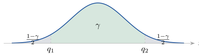
Фигура 13.1: Симетричен избор на квантилите. Защрихованата площ между q_1 и q_2 е нивото на доверие \gamma ; в двете опашки остава по \frac{1-\gamma}{2} . При симетрично около нулата разпределение q_1 = -q и q_2 = q .
