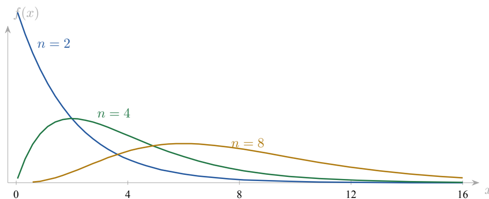
Фигура 9.1: Плътността на \chi^2(n) за три стойности на n . С растеж на n върхът се измества надясно и кривата се сплесква — очакването е n , а дисперсията 2n . Разпределението живее само върху положителната полуос (то е сума от квадрати) и е силно несиметрично при малки n ; точно затова доверителният интервал за дисперсията в лекция 13 се нуждае от два различни квантила, а не от \pm q както при нормалното.
