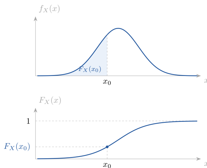
Фигура 8.1: Непрекъснати аналог на стъпаловидната функция от фигурата в лекция 5 . Гор е плътността f_X ; заштрихованата площ вляво от x_0 е \mathbb{P}(X < x_0) . Долу е функцията на разпределение F_X : нейната височина в x_0 е точно тази площ. Скоковете от дискретния случай са изгладени — F_X е непрекъсната, а наклонът ѝ във всяка точка е стойността на плътността там.
