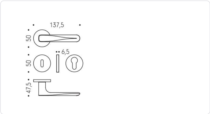
DISEGNO QUOTATO · MISURE IN MM
