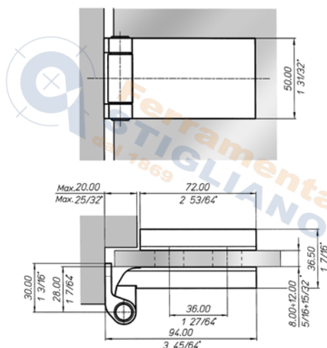
GAHA1L6D Braccio Lungo (+ mm 5,5) Long Arm (+ mm 5,5)
