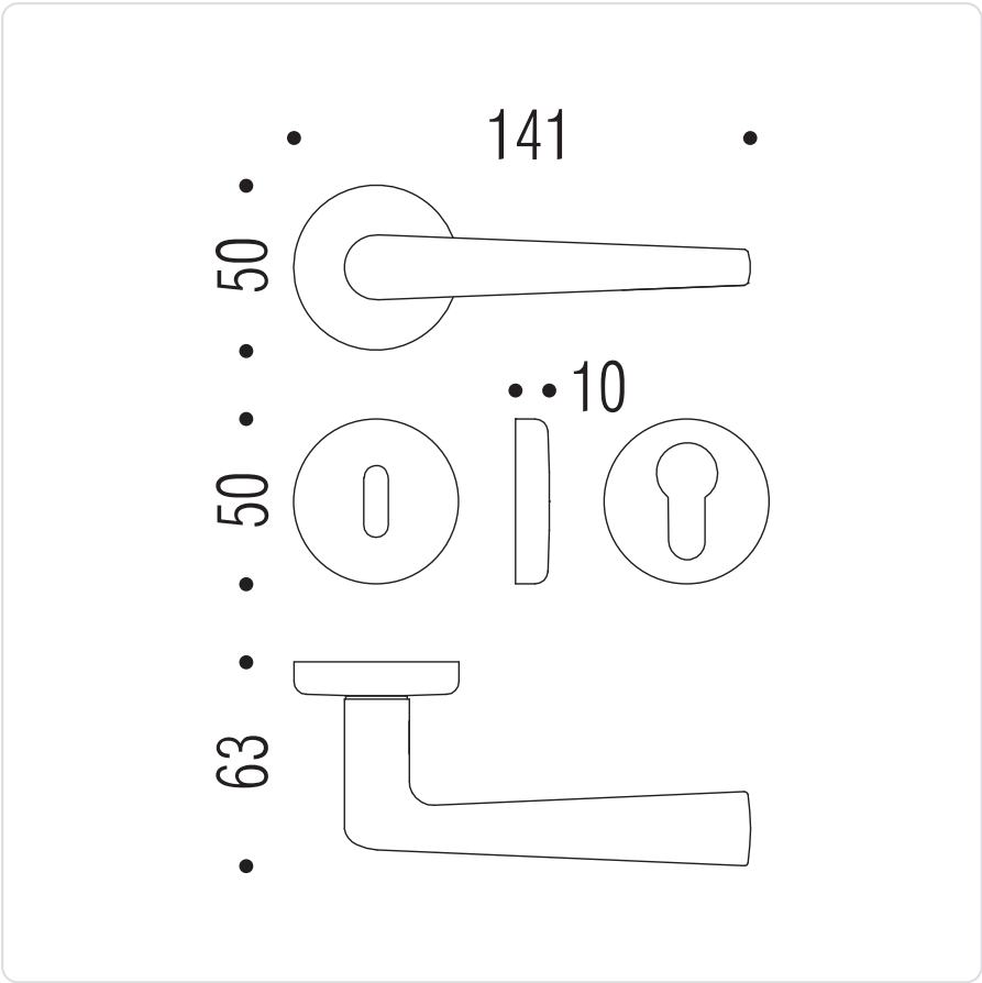
DISEGNO QUOTATO · MISURE IN MM
