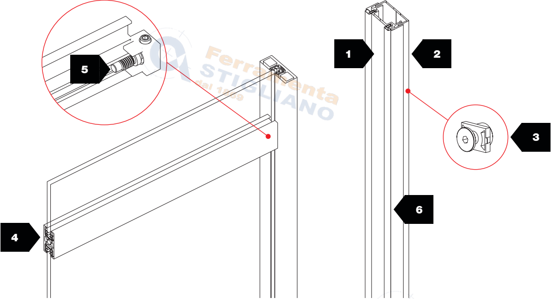
ADJUSTABLE CLOSING JAMB BATTUTA LATERALE REGOLABILE
