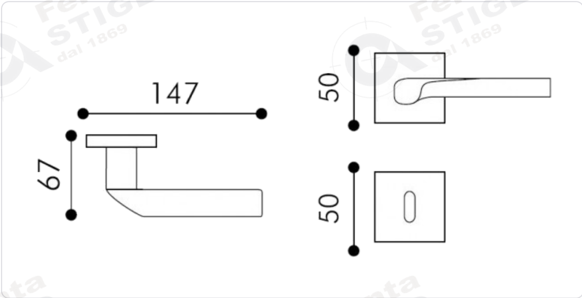
DISEGNO QUOTATO · MISURE IN MM
