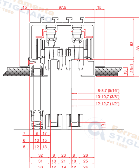
DOUBLE DOOR + FIXED GLASS / PORTA DOPPIA + FISSO
