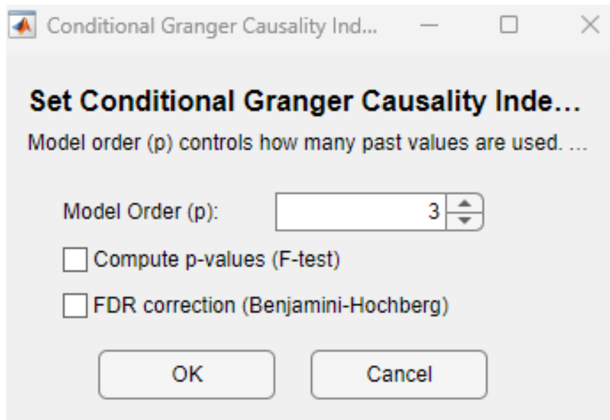
Σχήμα 4.8: Παράθυρο παραμέτρων του Δείκτη Δεσμευμένης Αιτιότητας κατά Granger
