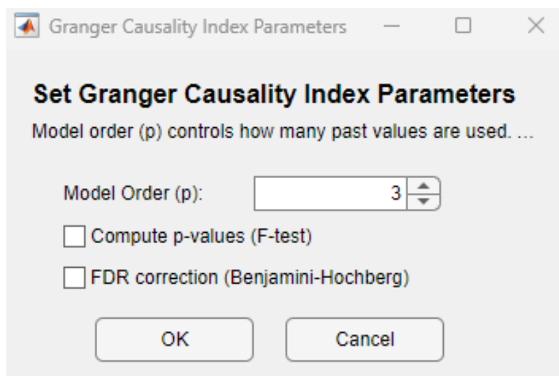
Σχήμα 4.7: Παράθυρο παραμέτρων του Δείκτη Αιτιότητας κατά Granger
