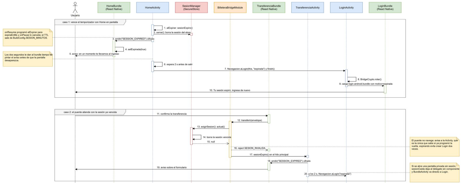
Figura 3. Expiración de la sesión por temporizador y por rechazo del puente
