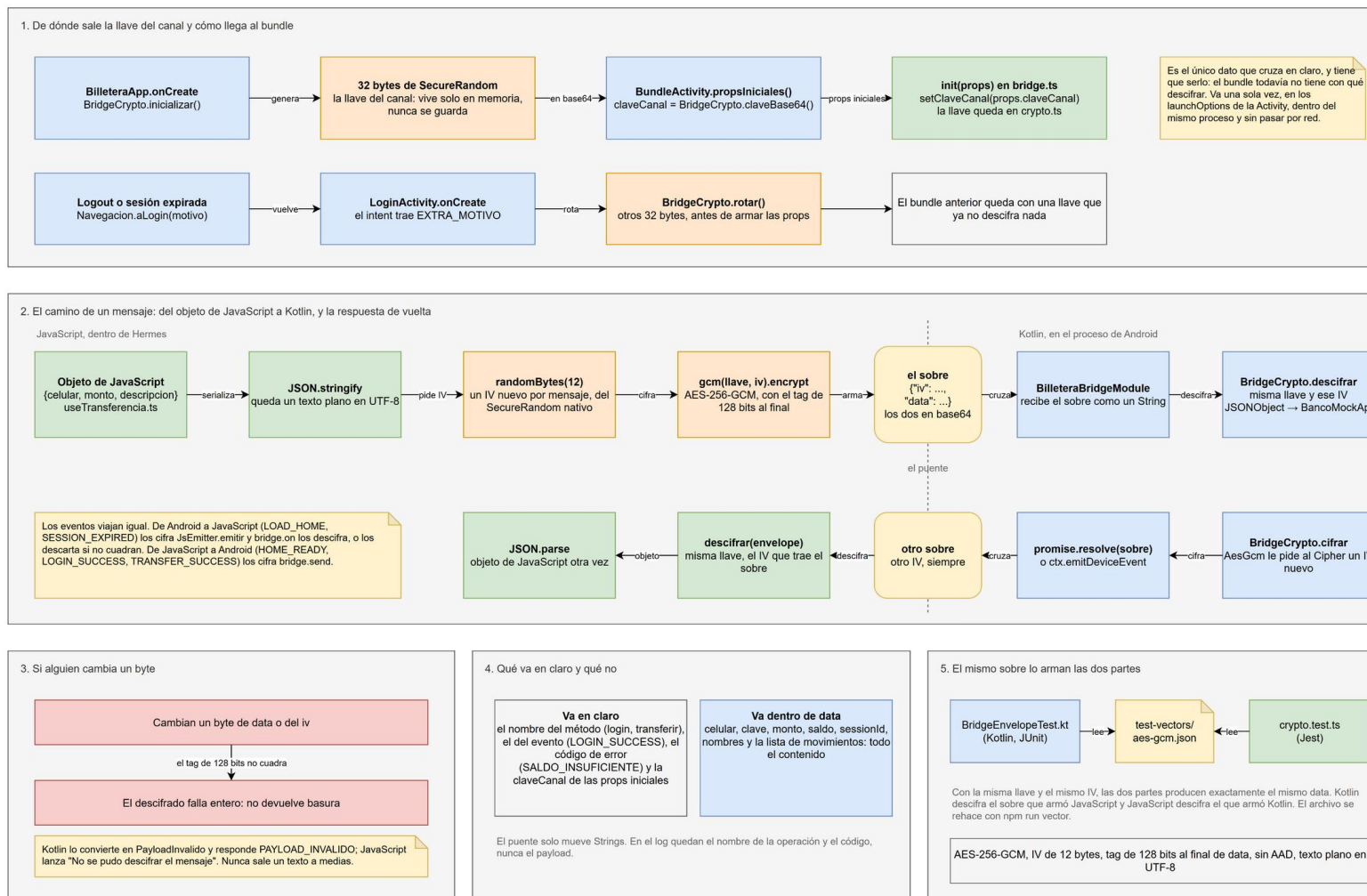
Figura 4. El sobre AES-256-GCM que envuelve todo lo que cruza el puente
