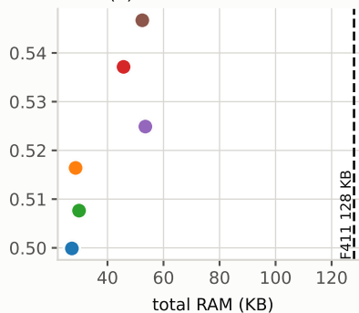
(d) int8 AUPRC vs SRAM
