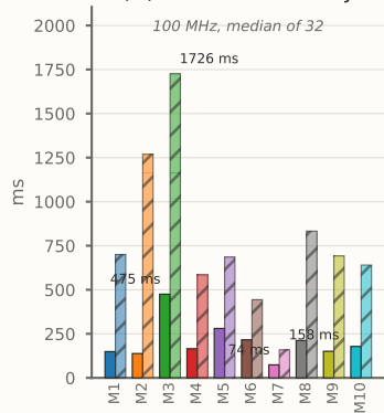
(D) Measured latency
