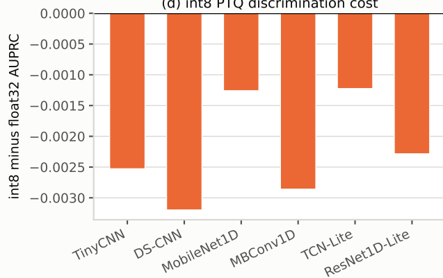
(d) int8 PTQ discrimination cost
